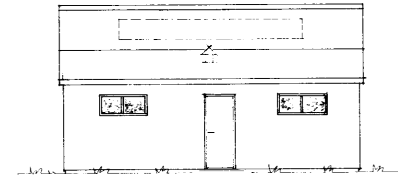
SÚÐURHLÍÐ
