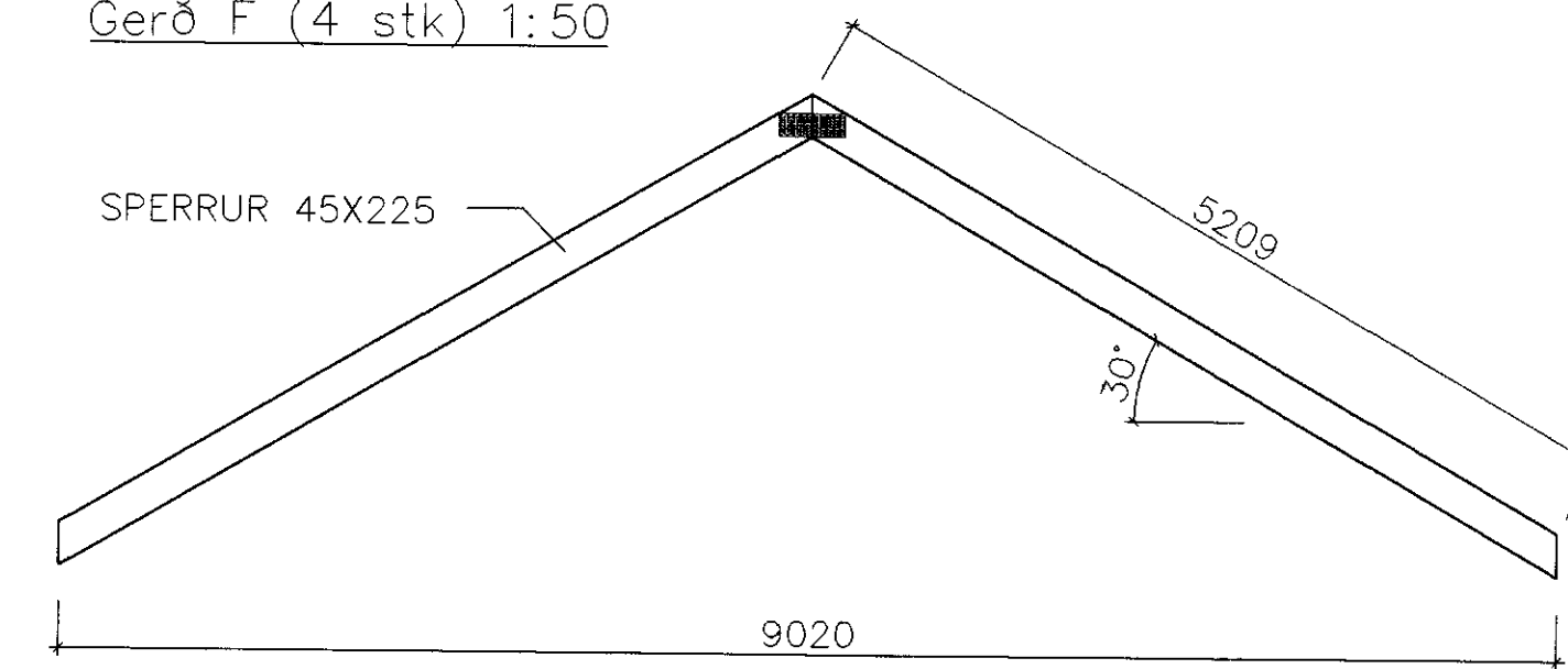
Gerð F (4 stk) 1:50
