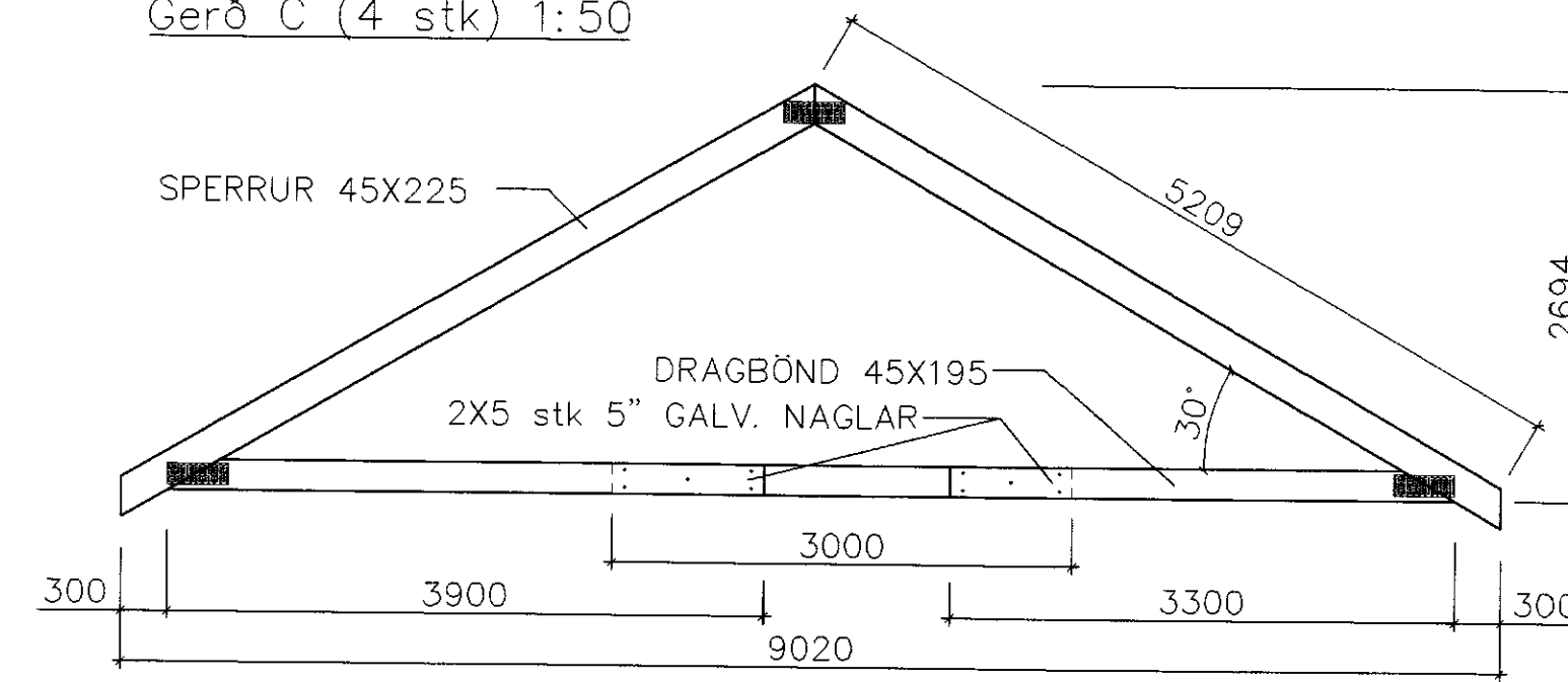
Gerð C (4 stk) 1:50
