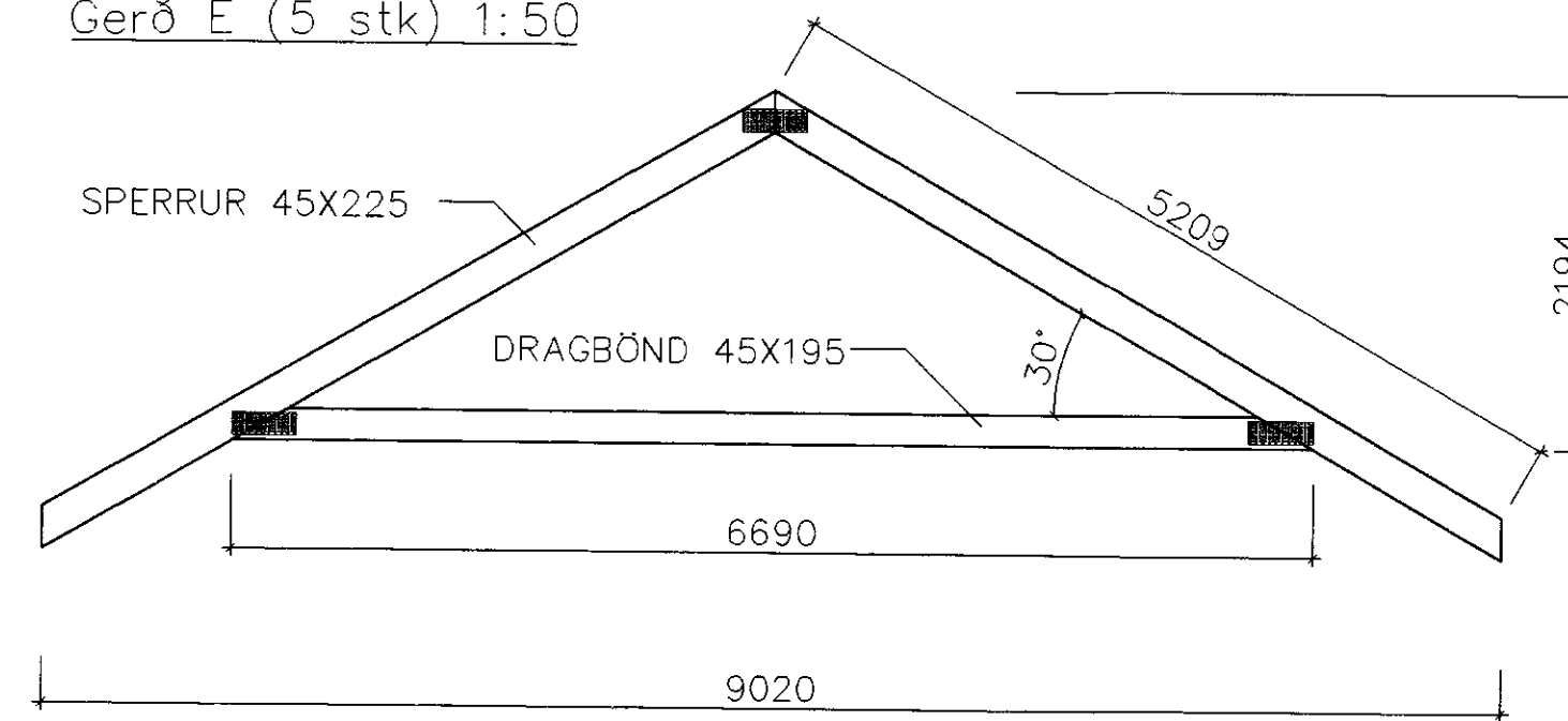
Gerð E (5 stk) 1:50
