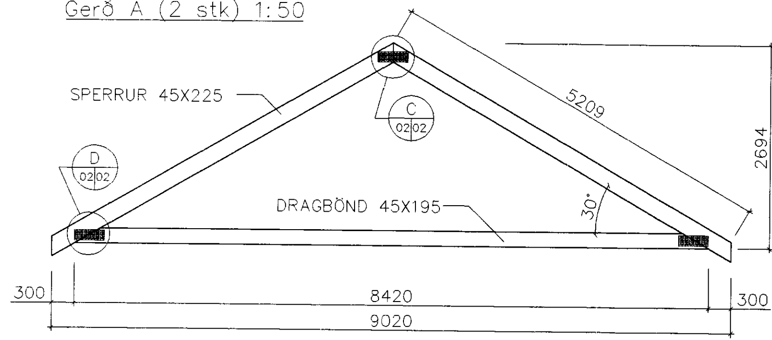
Gerð A. (2 stk) 1:50
