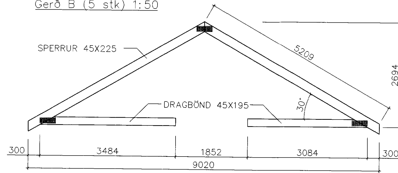
Gerð B (5 stk) 1:50
