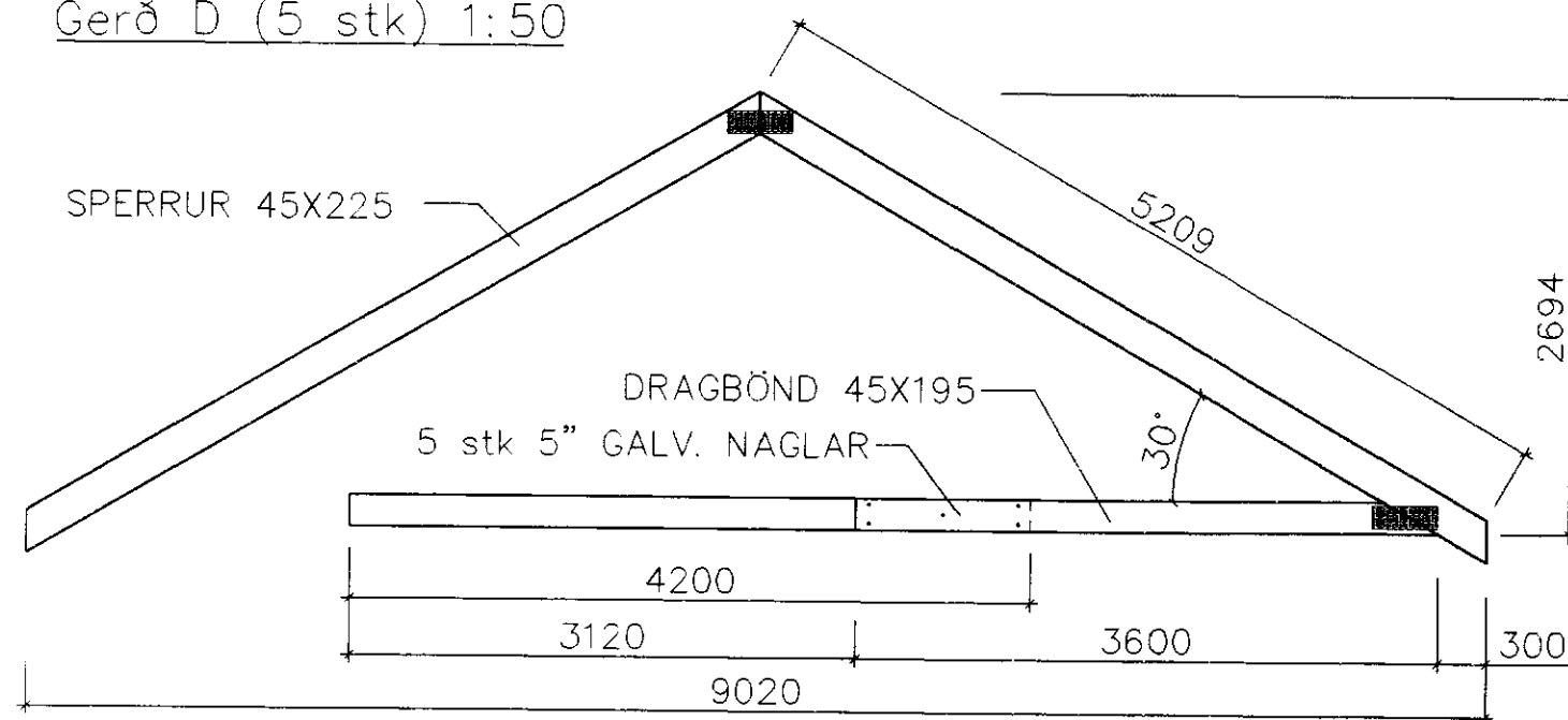
Gerð D (5 stk) 1:50
