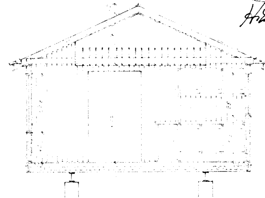
SNEIÐING 1:50
