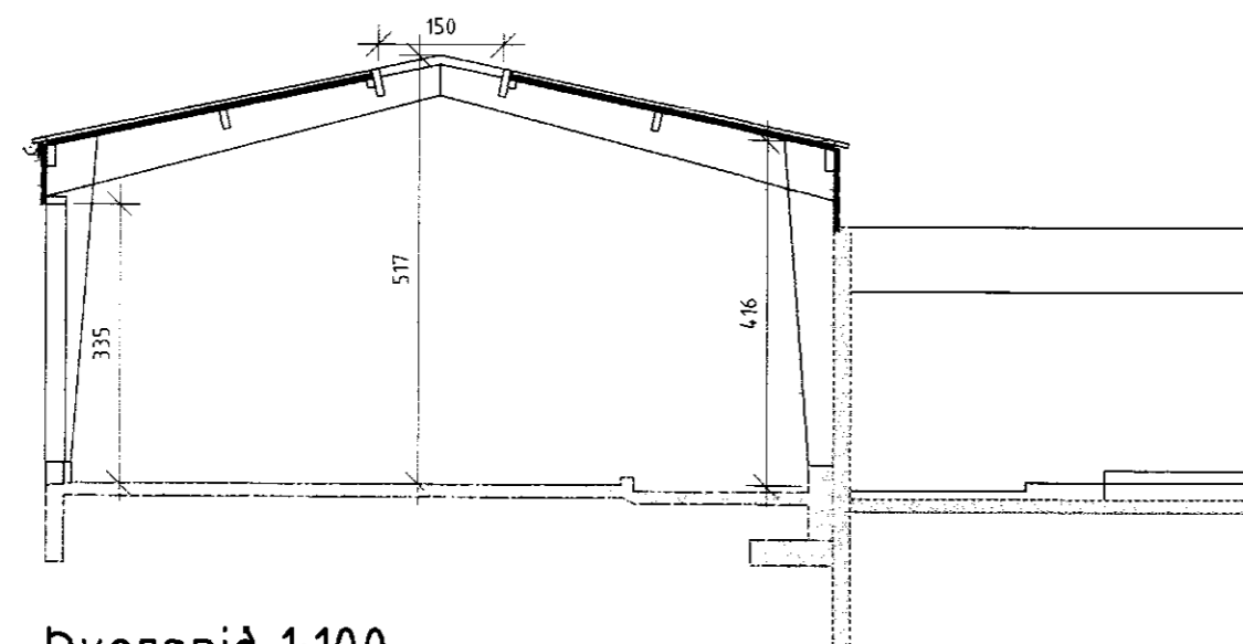
Þversnið 1:100
