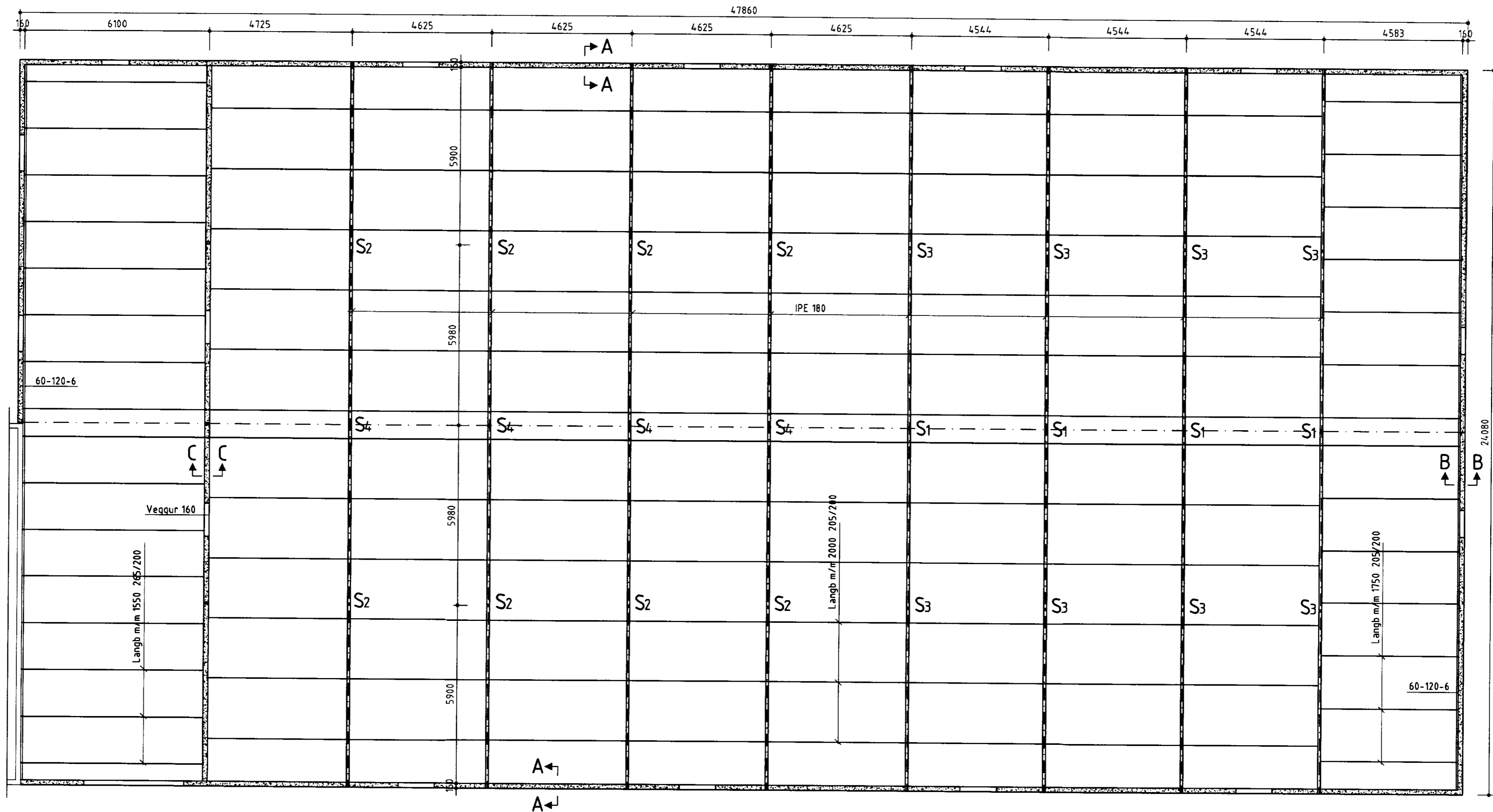
Grunmynd af þaki Mkv. 1:100
