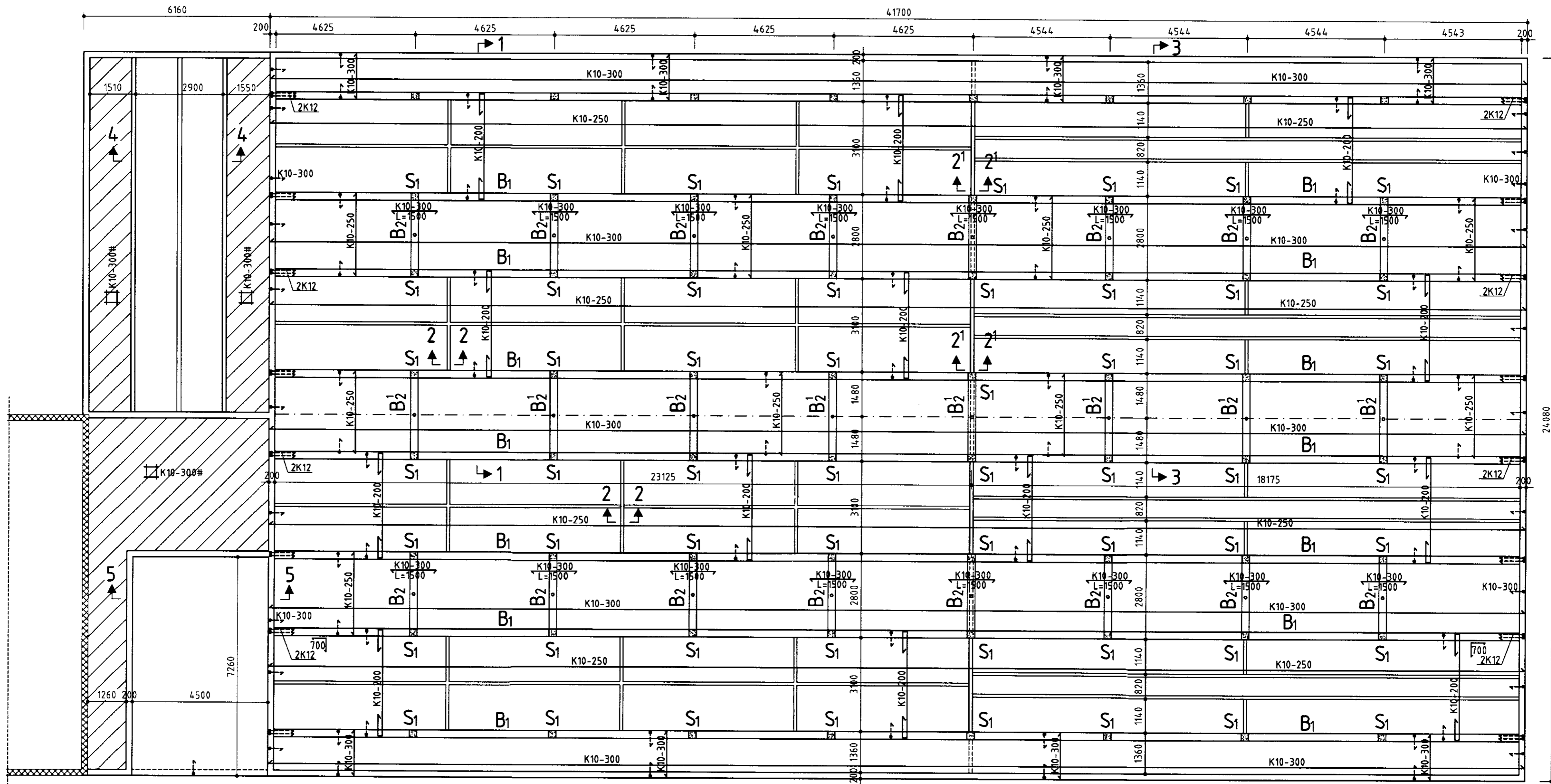
Grunnmynd Mkv. 1:100
