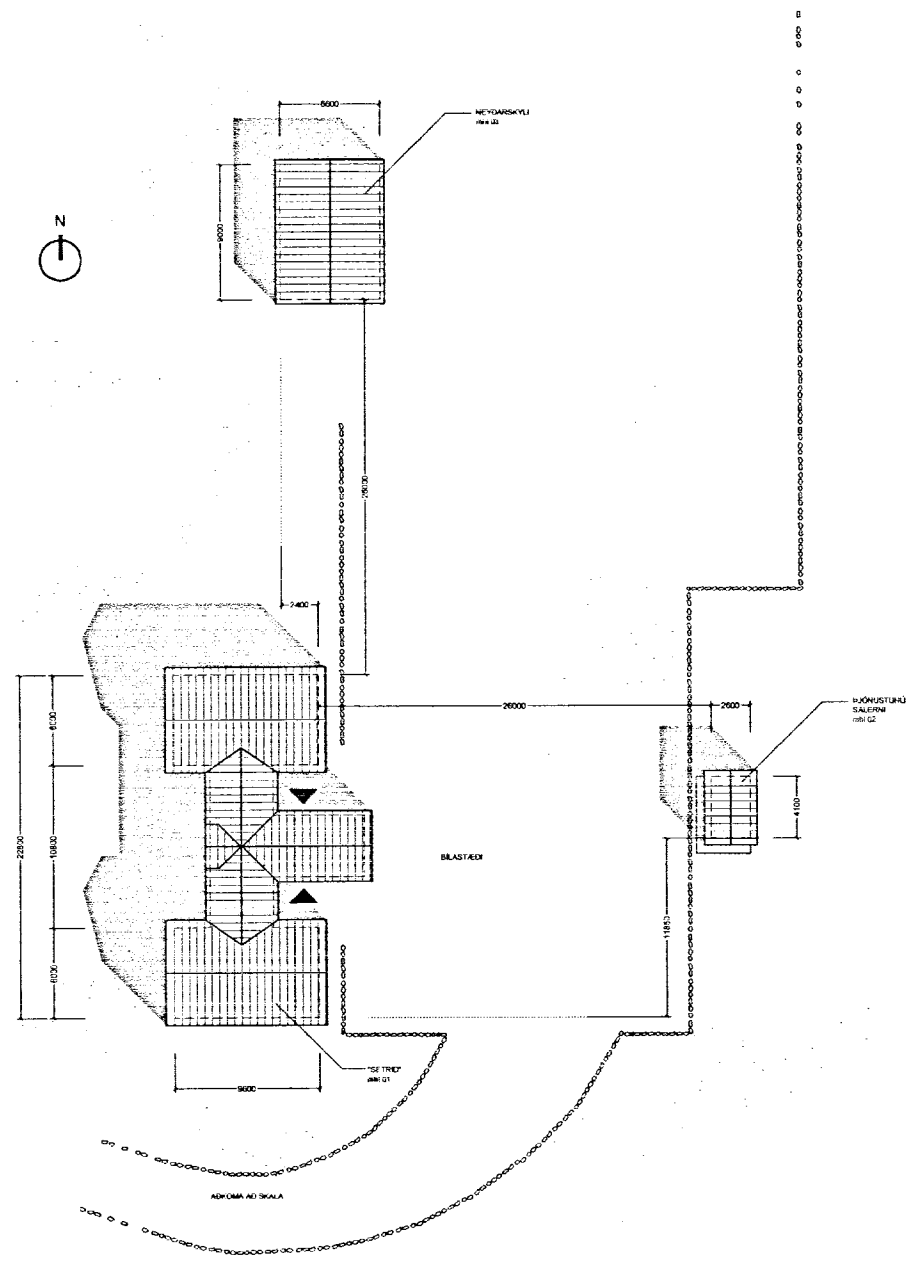
AFSTÖÐUMYND M 1:500
