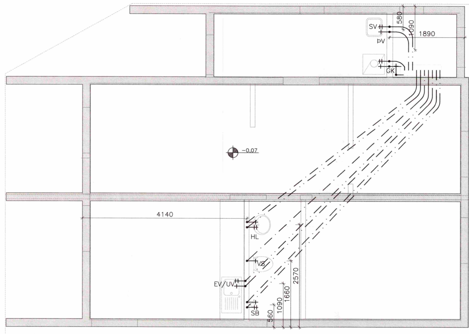
GRUNNMYND NEYSLUVATNSLAGNA Mkv. 1:50
