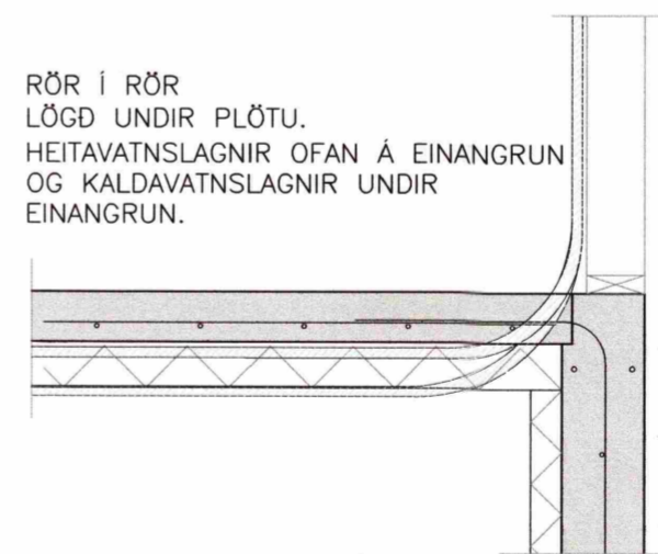
STAÐSETNING STÚTA VIÐ ÚTVEGG OG UNDIR PLÖTU Mkv. 1:20
