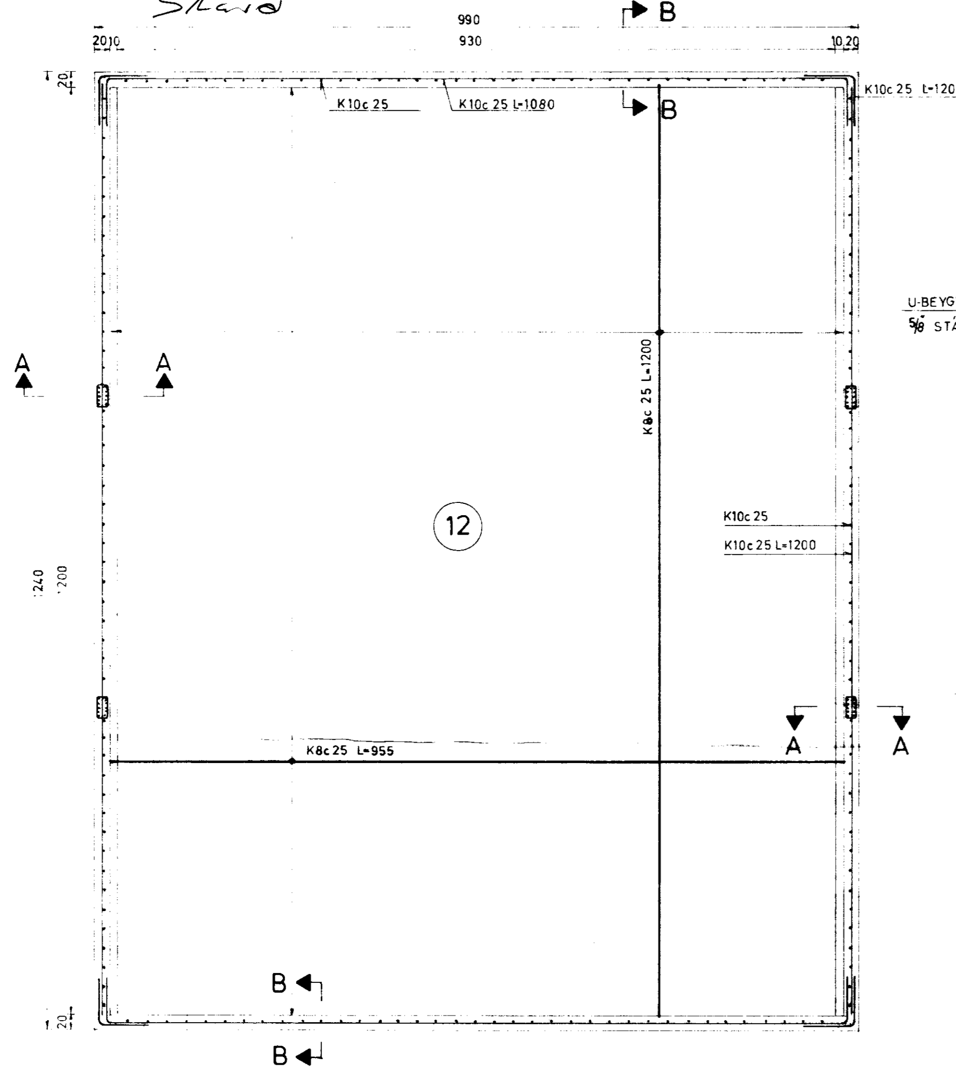
GRUNNMYND 1:50
