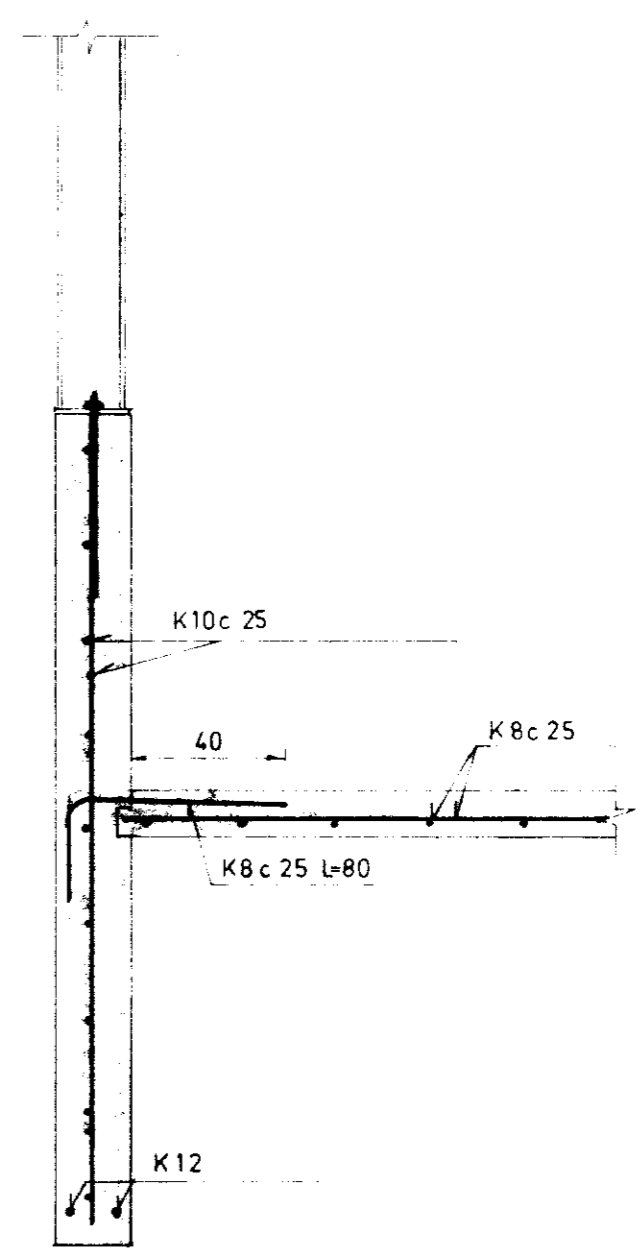
SNID B-B 1:20
