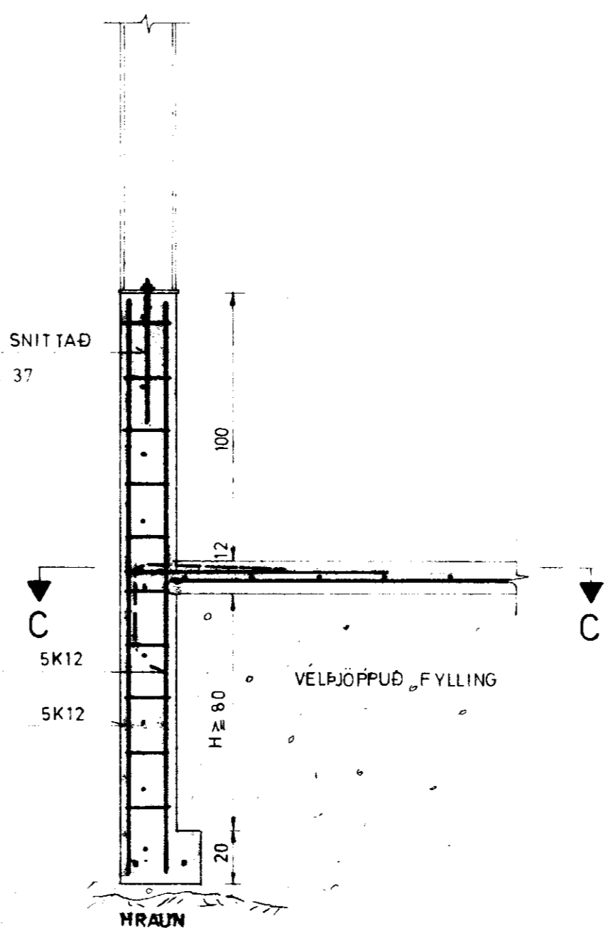
SNID A-A 1:20
