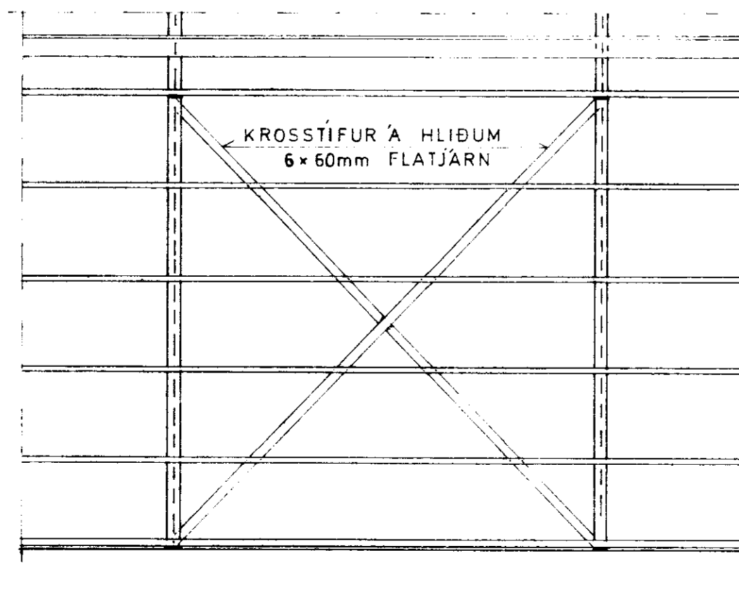
KROSS-STÍFUR SJÁ STADSETNINGU Á BL.NR. 2. MKV, 1:50
