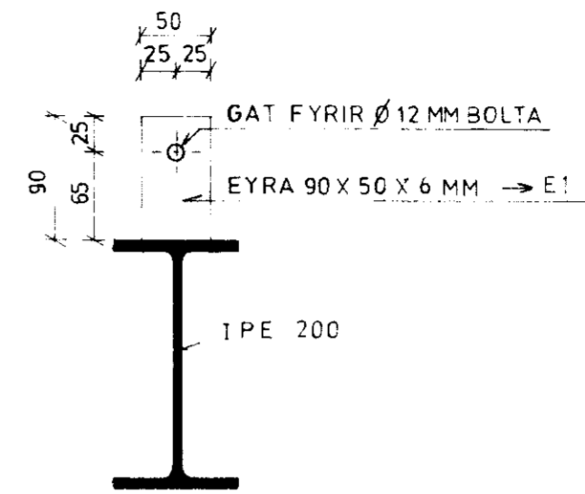
EYRU FYRIR ÞAKBITI 2" x 7" MK L, 1:50
