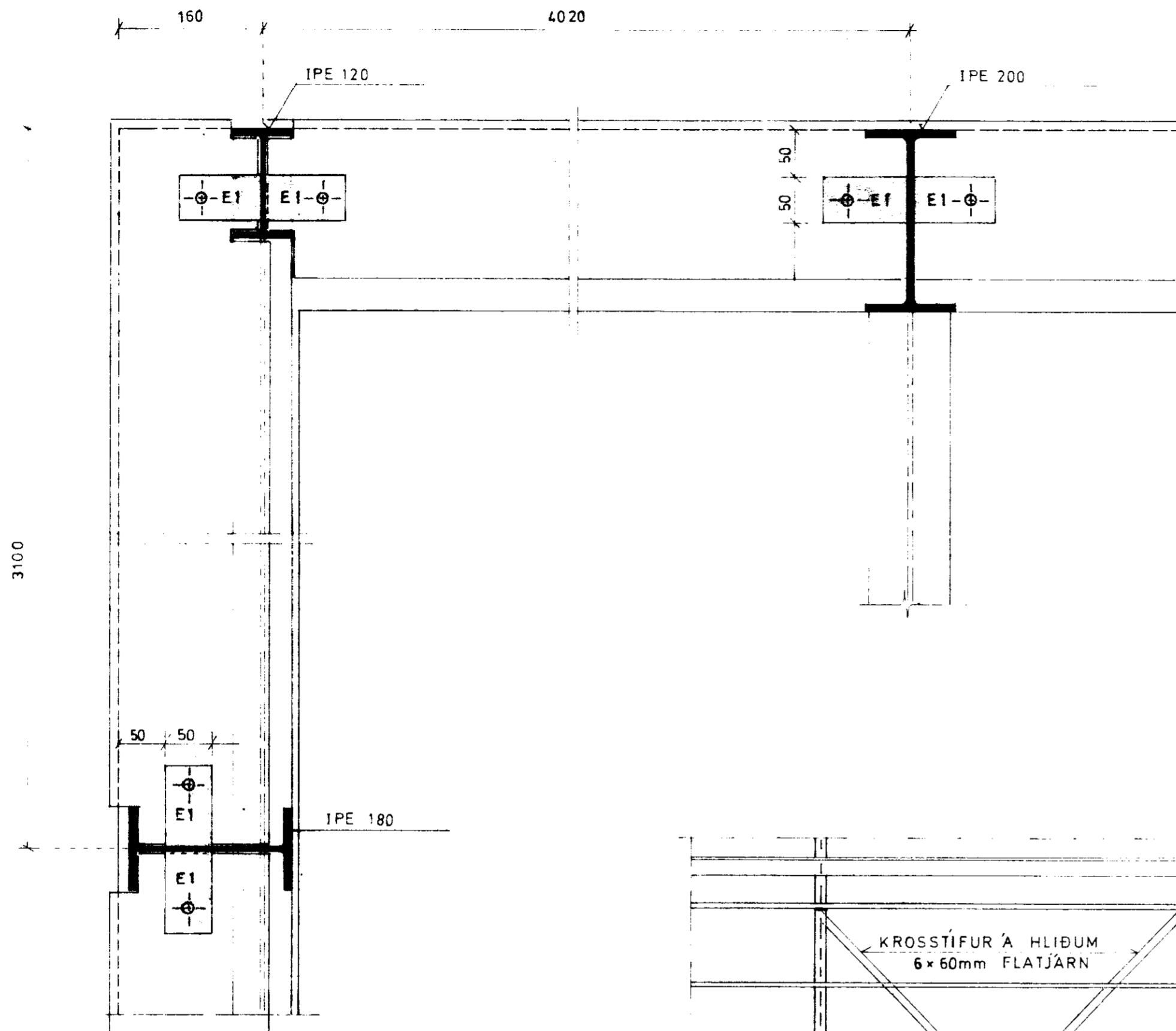
STADSETNING STÁLRAMMA, EYRA OG BITAR (2" x 7") Á HLIÐUM MKV, 1:50
