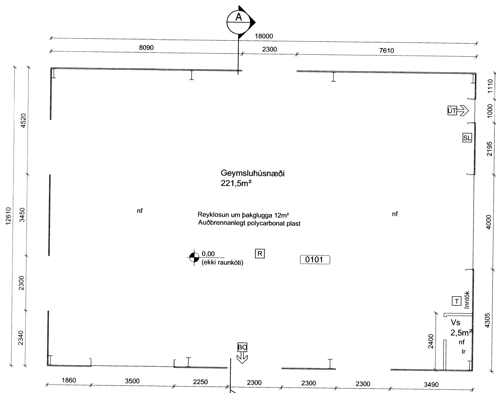
Grunnmynd M 1:100
