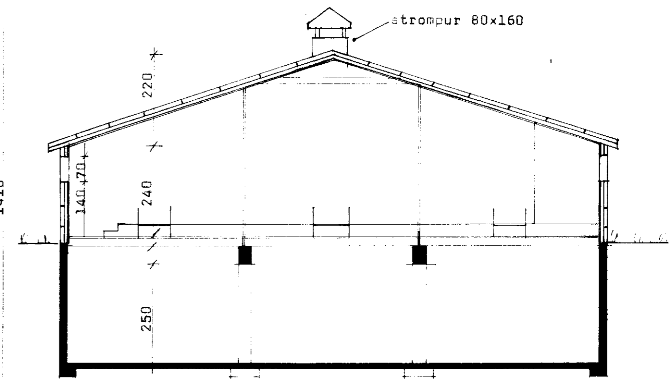
Skurður
