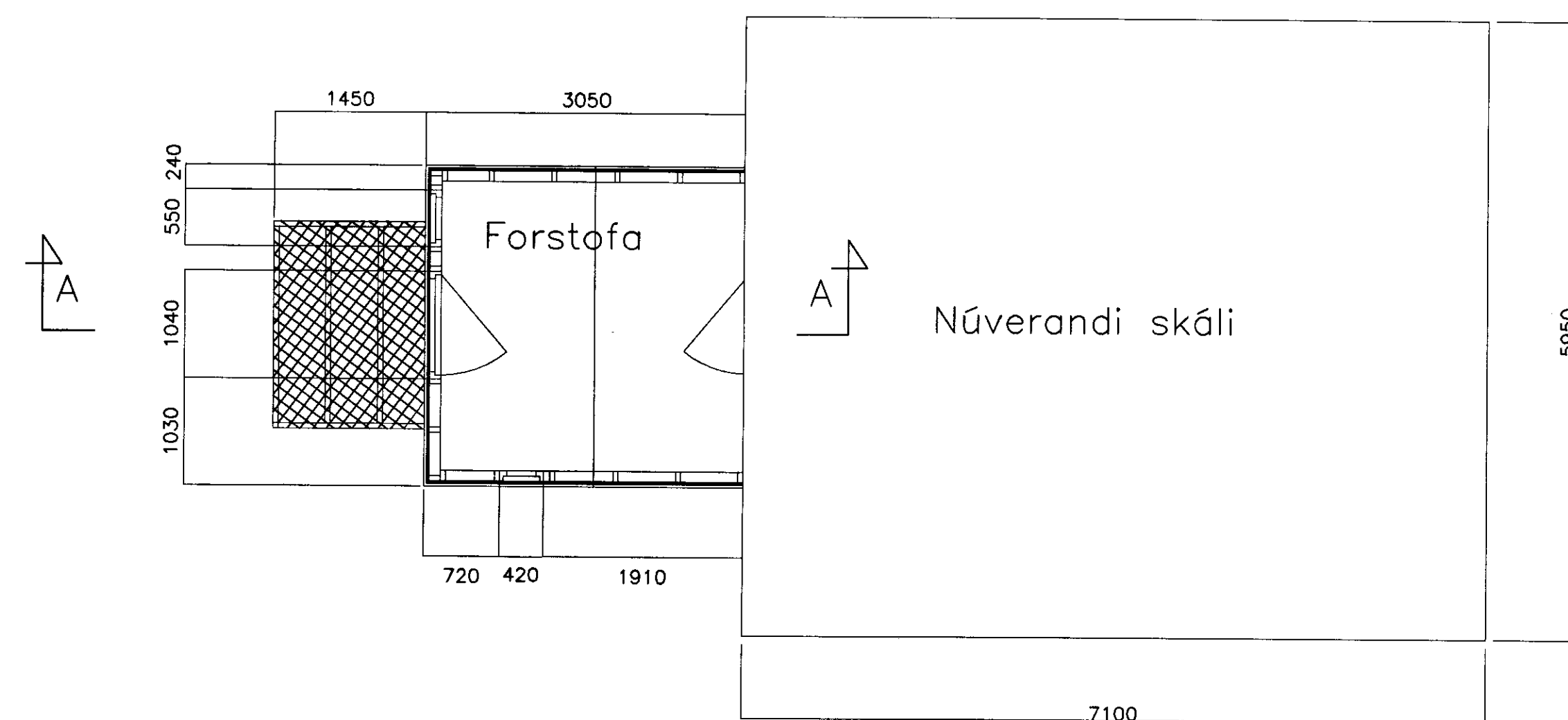
Snið A-A 1:50
