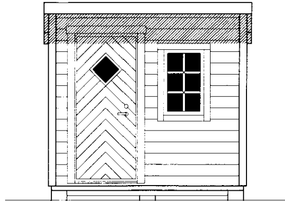
FASAD FRAMSIDA
