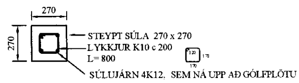
SNID G-G 1:20
