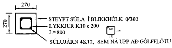
SNID G-G 1:20
