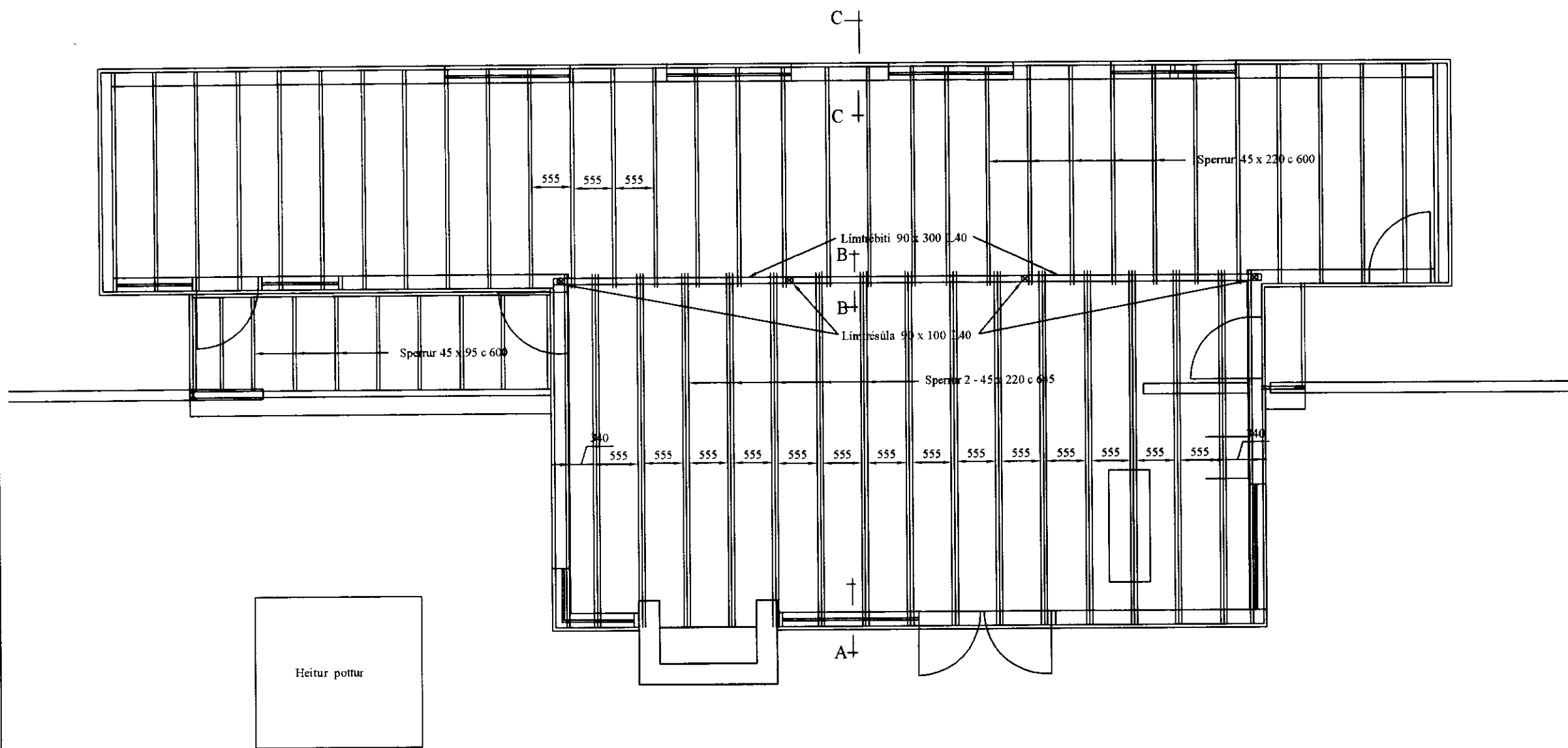
GRUNNMYND 1:50
