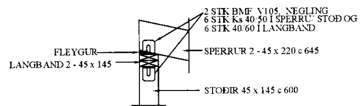
SNID A-A 1:20
