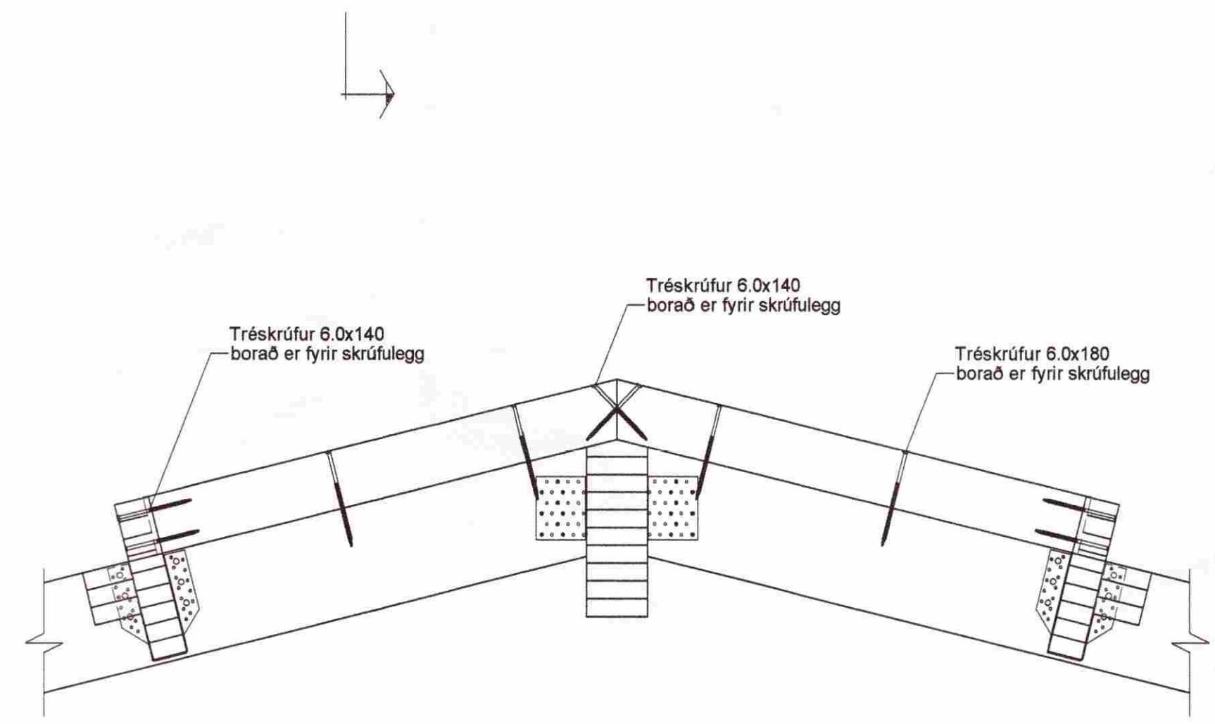
Þversnið D Mkv. 1:10 101
