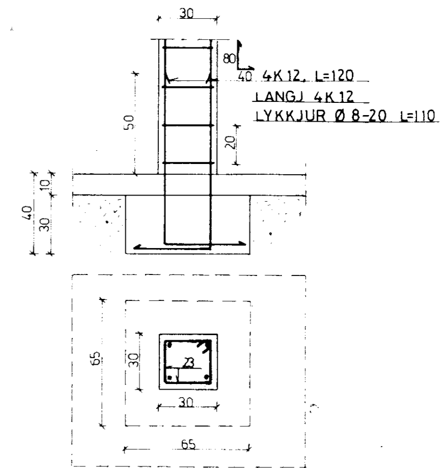
STOÐ MED UNDIRST. M. 1:20
