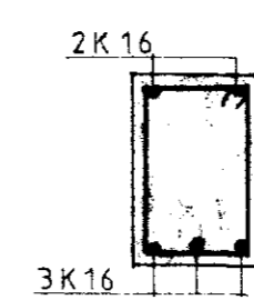
C-C M=1:20
