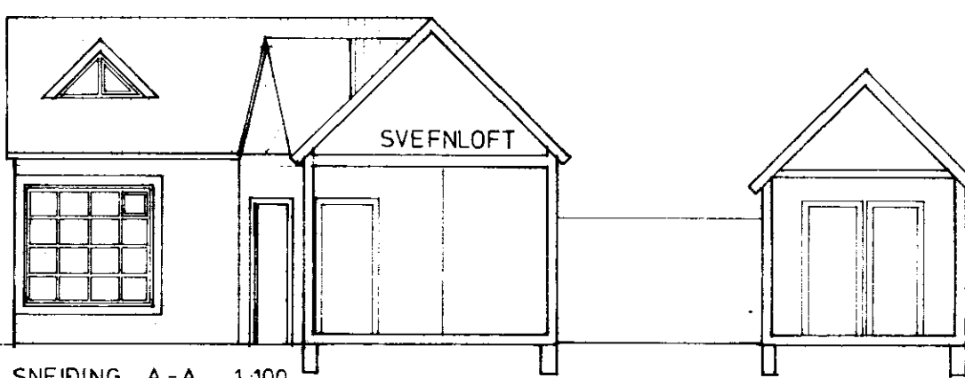
SNEIDING A-A 1:100
