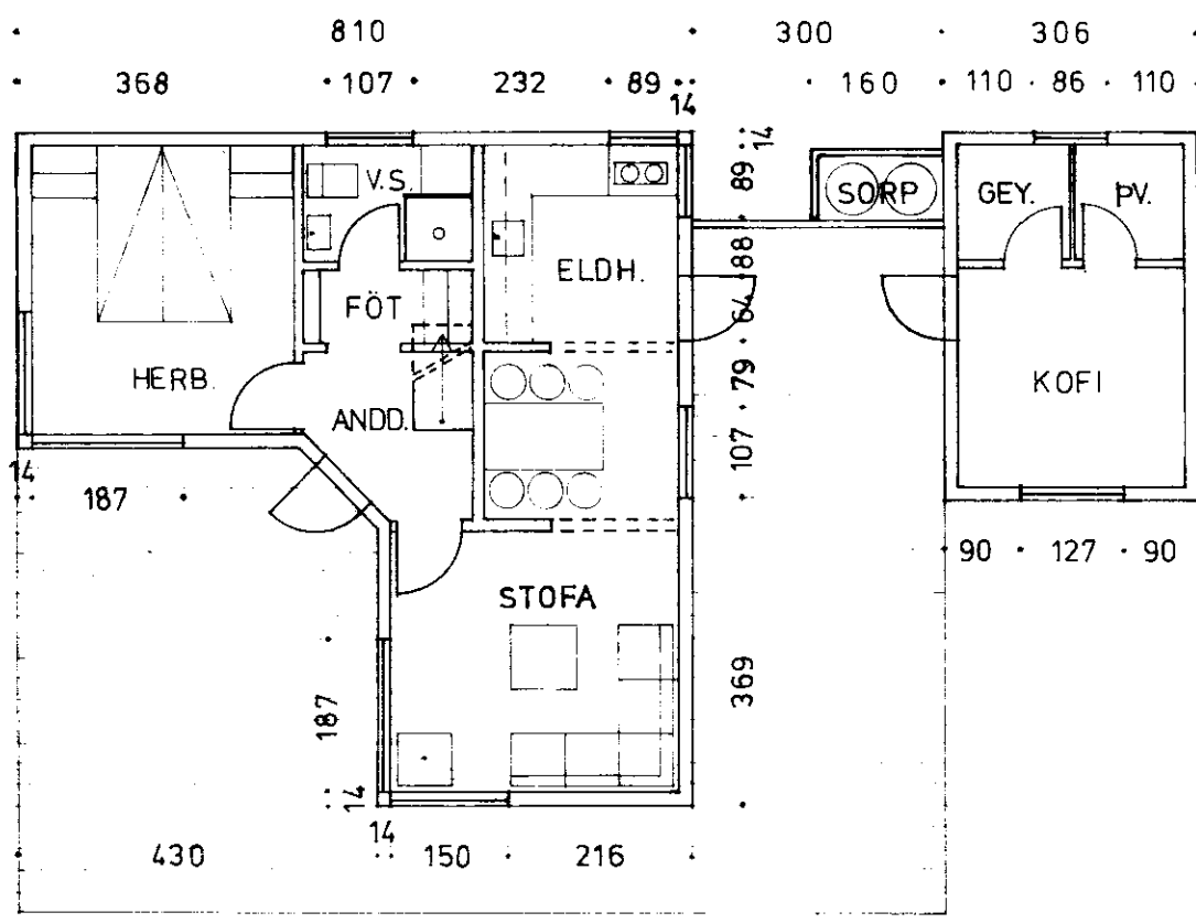
GRUNNMYND 1:100
