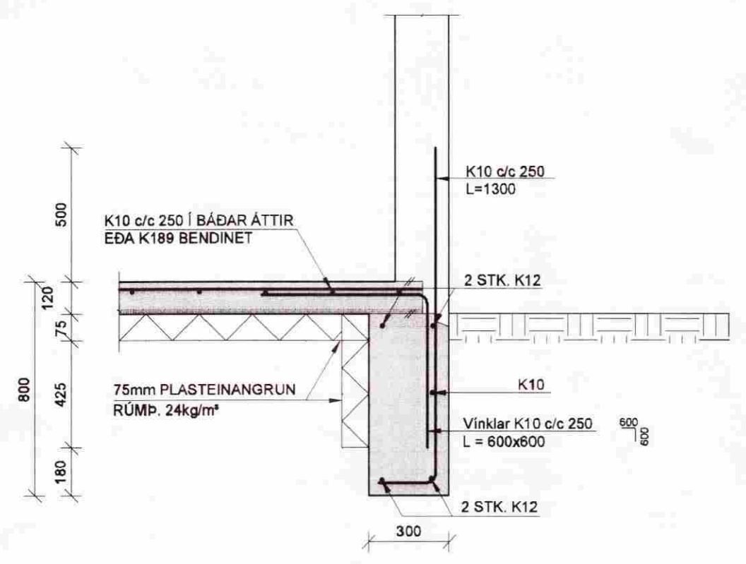
SNÍÐ A 1:20 B2-1
