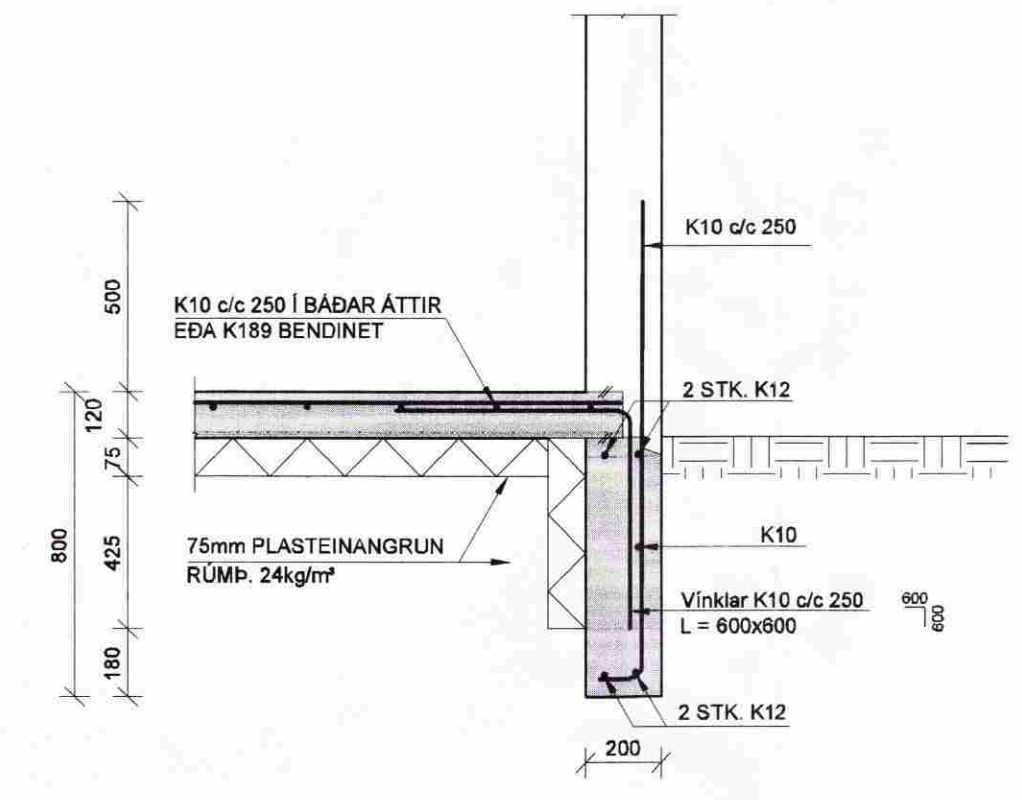
SNÍÐ I 1:20 B2-1
