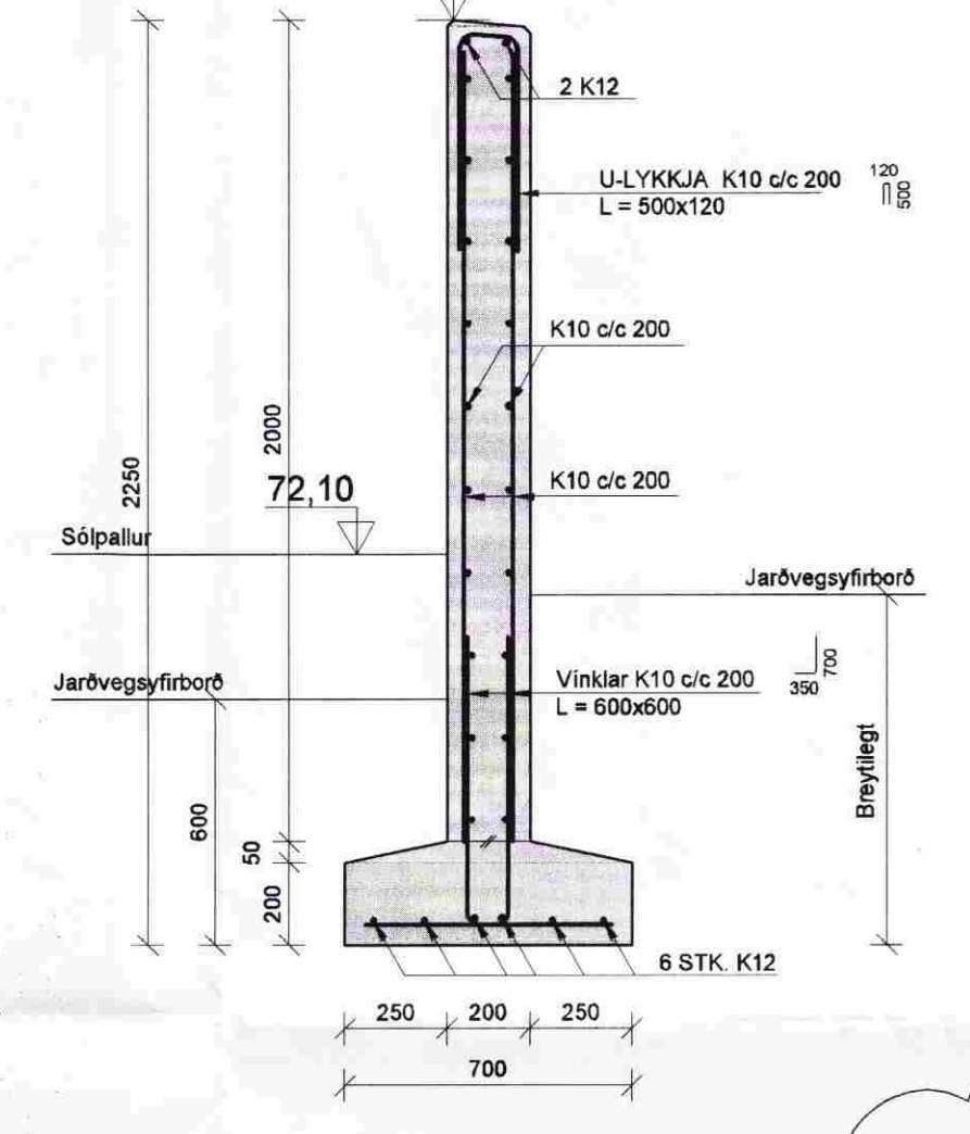
SNÍÐ H 1:20 B2-1
