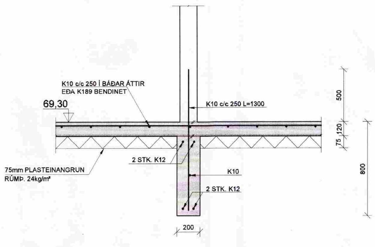
SNÍÐ C 1:20 B2-1
