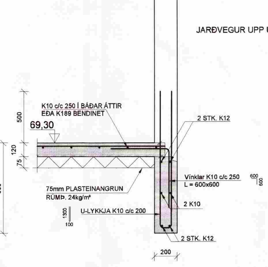
SNÍÐ B 1:20 B2-1
