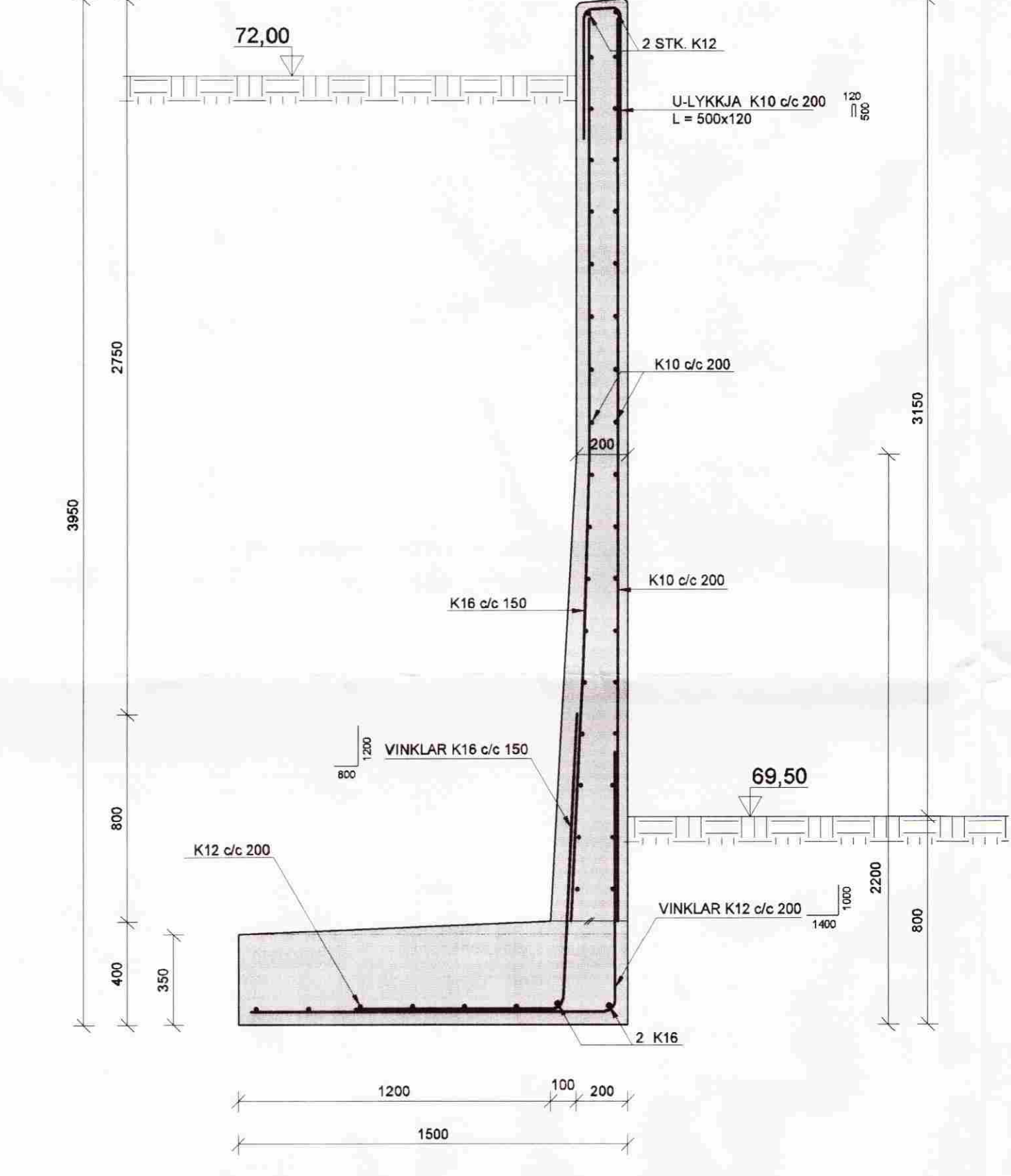
SNÍÐ J 1:20 B2-1
