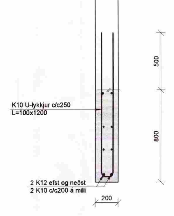
SNÍÐ E 1:20 B2-1
