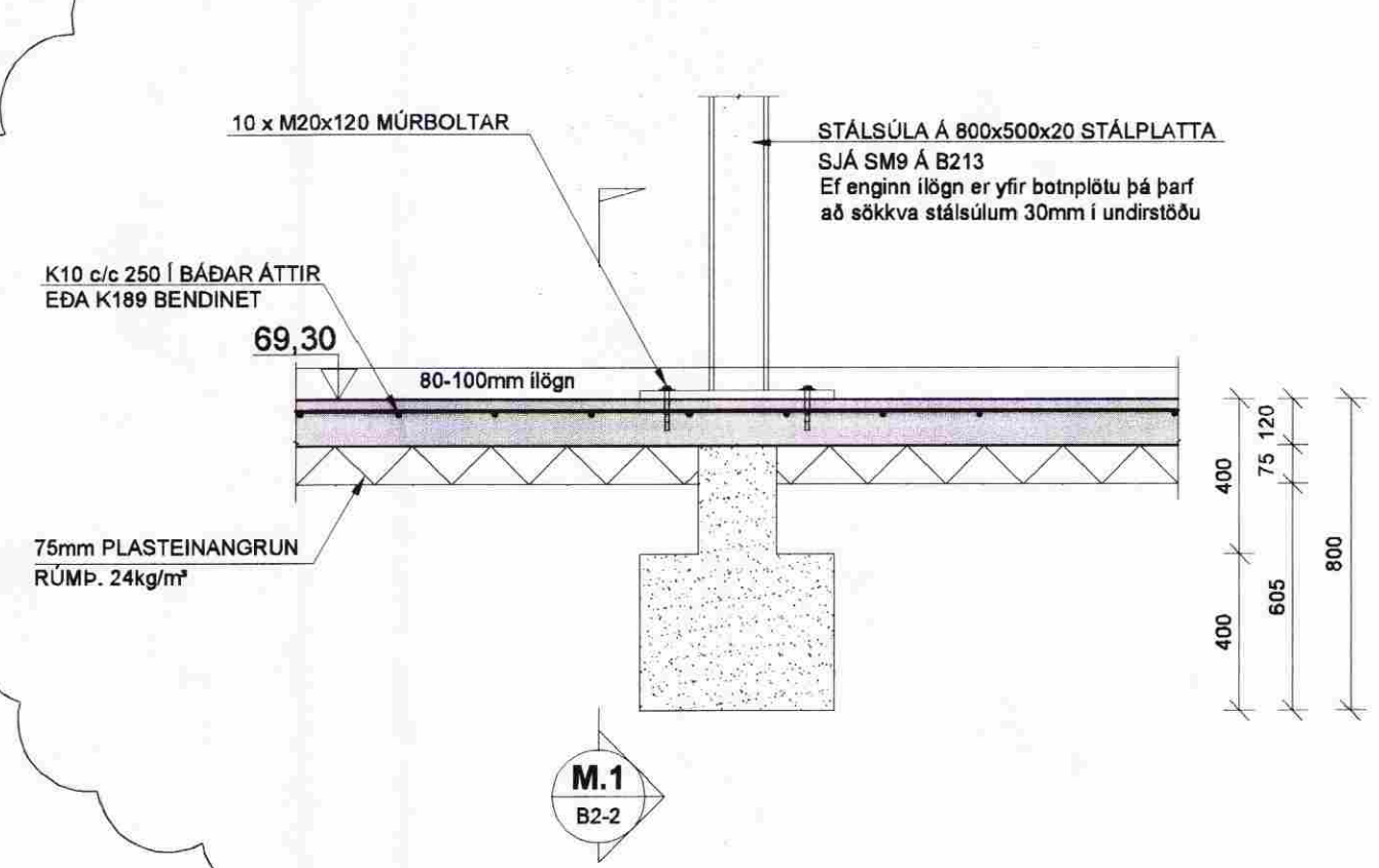
SNÍÐ M 1:20 B2-1
