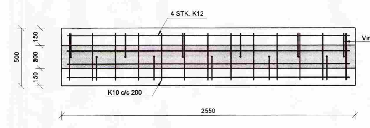
SNÍÐ J1 1:20 B2-2
