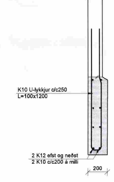
SNÍÐ D 1:20 B2-1
