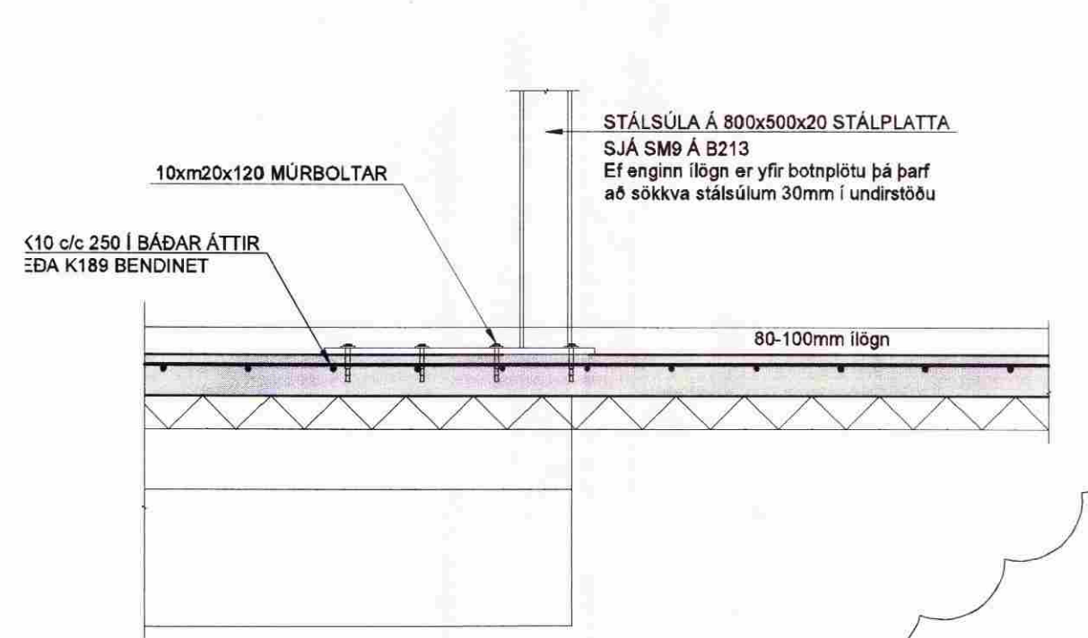
SNÍÐ M.1 1:20 B2-2
