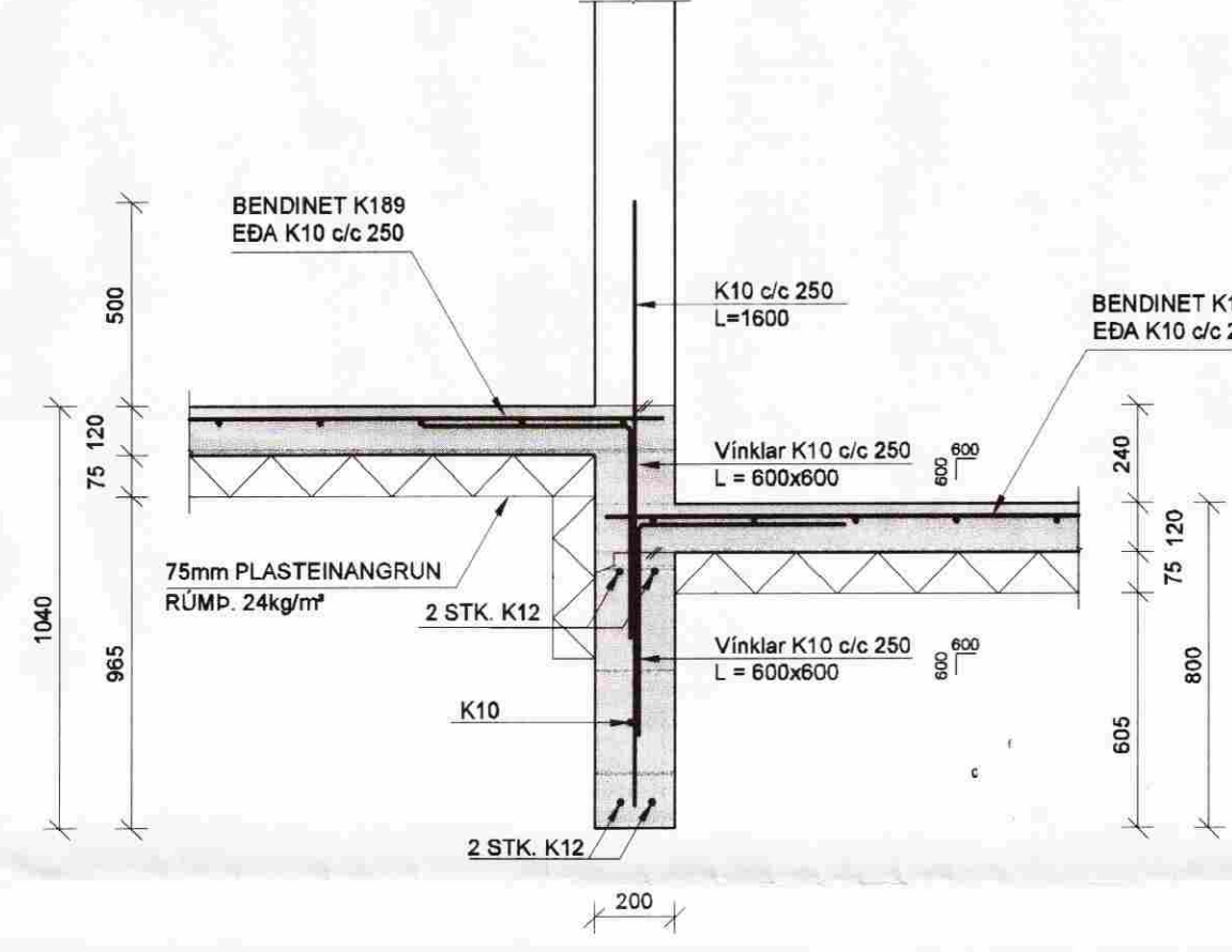
SNÍÐ G 1:20 B2-1
