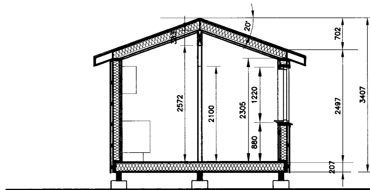
SNID A-A MKV.2
