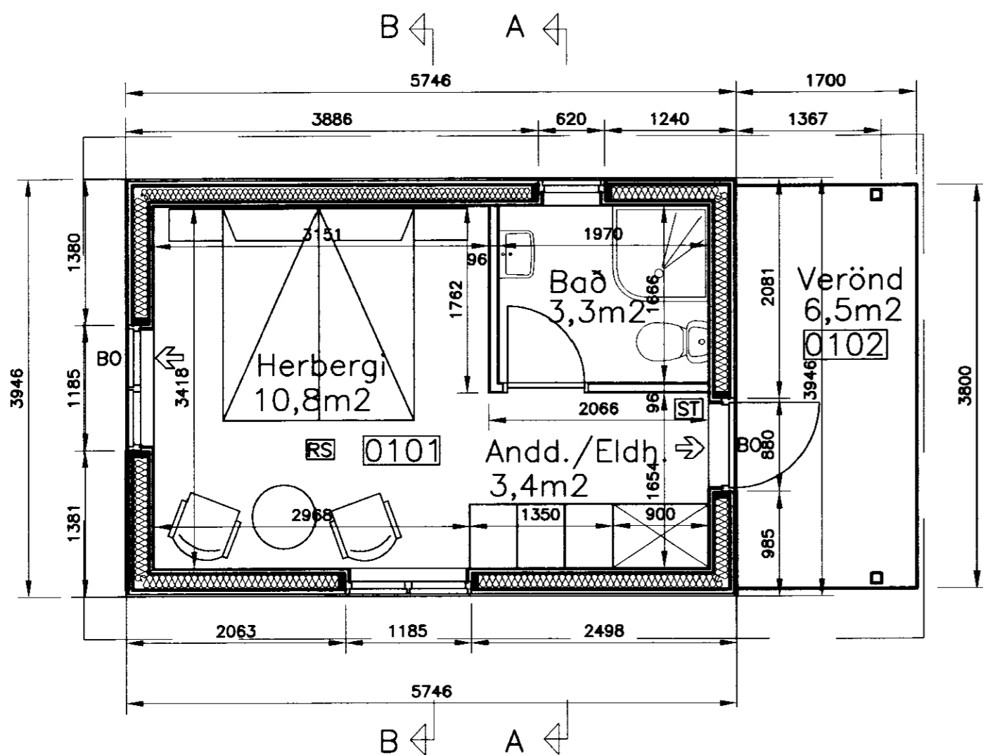
GRUNNMYND MKV.2
