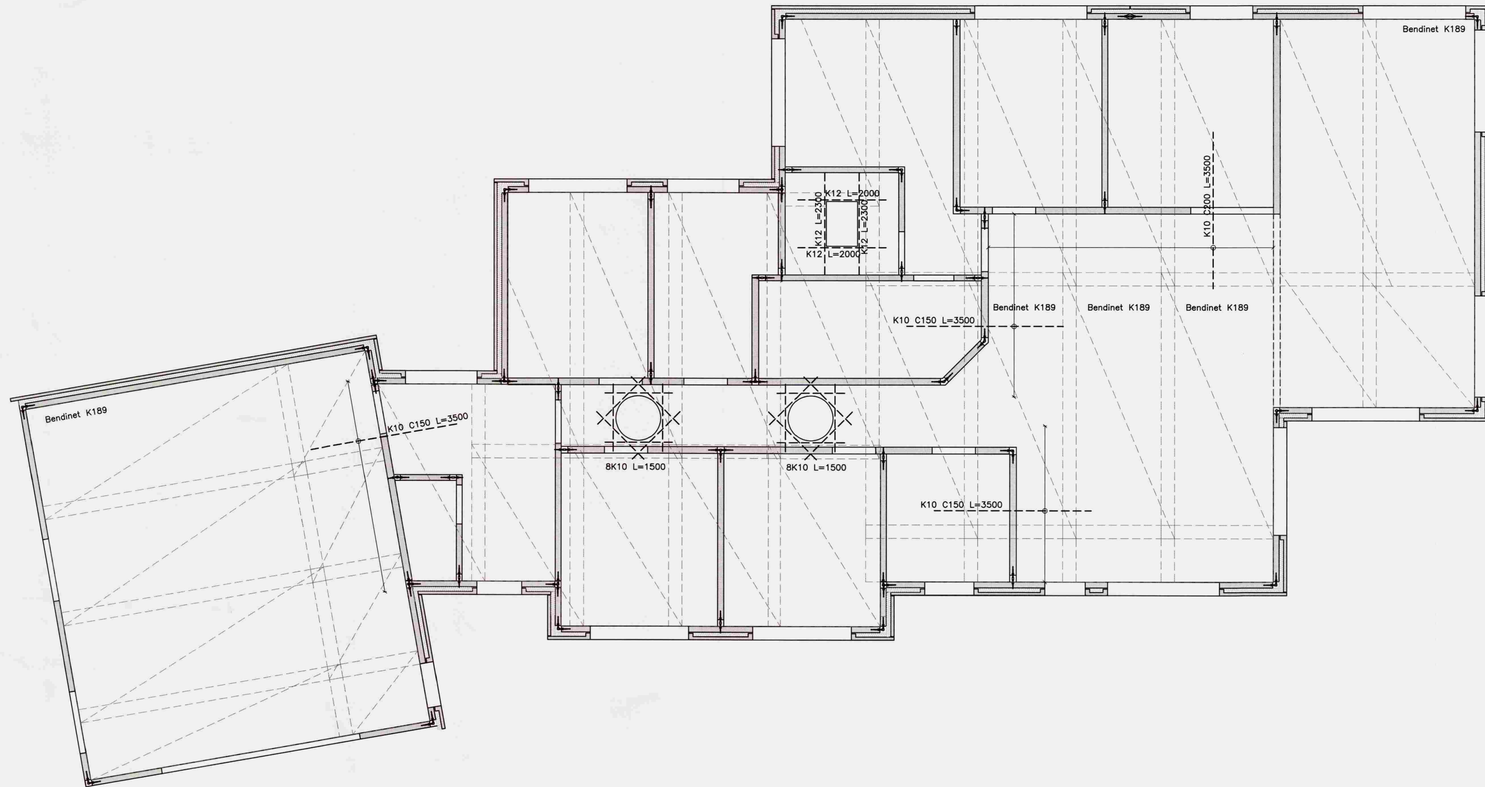
Járnabending, efri brún 1:50
