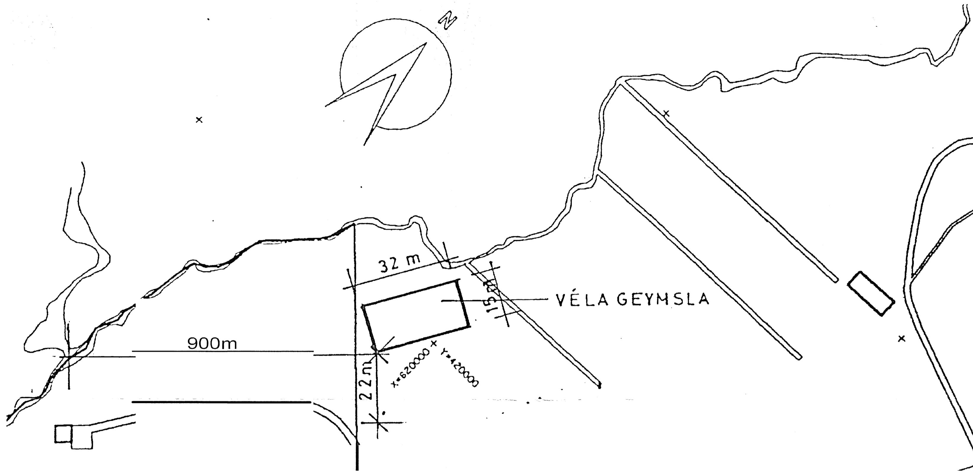
AFSTÖÐUMYND 1:500
