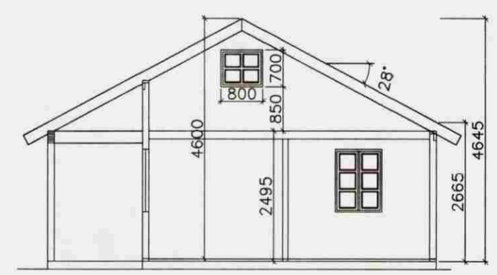
SNIÐ AA
