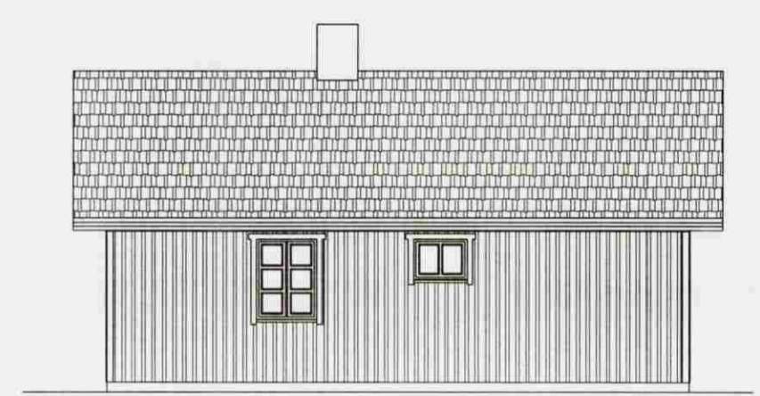
NORÐUR HLIÐ
