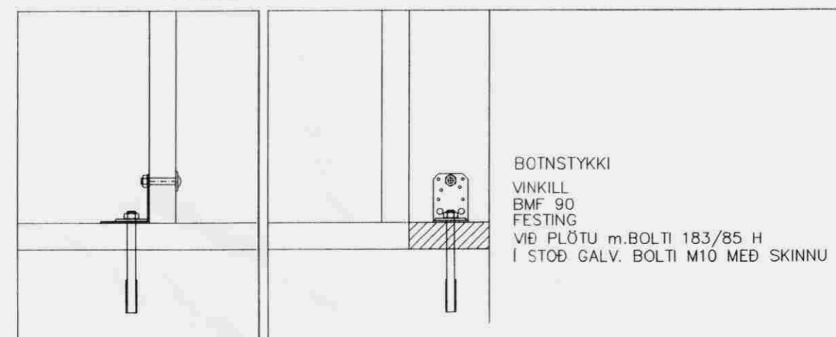
SÉRMYND FESTING VIÐ BOTNSTYKKI
