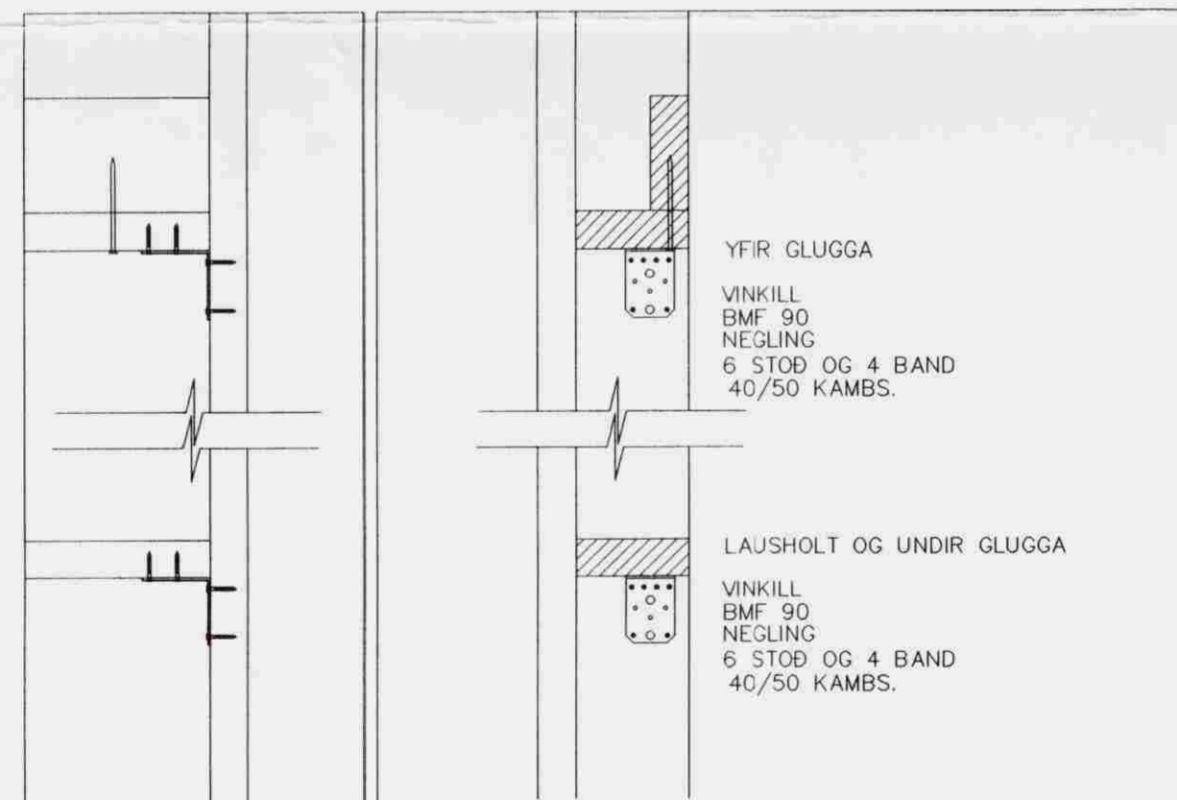
SÉRMYND FESTING YFIR OG UNDIR GLUGGA
