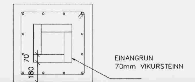
SKORSTEINN 1:20
