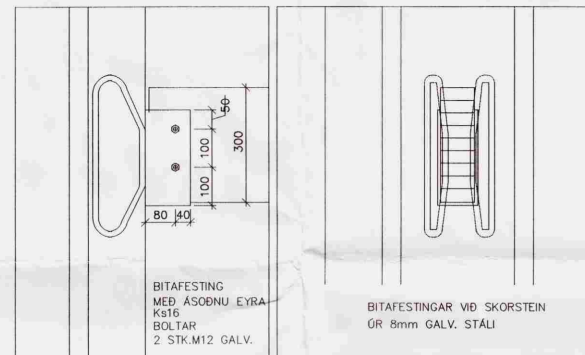
SÉRMYND FESTING LÍMTRÉS VIÐ SKORSTEIN
