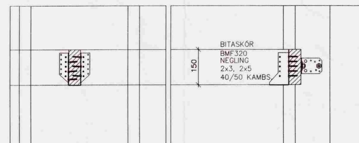
SÉRMYND FESTING GÓLFBITA VIÐ ÚTVEGG
