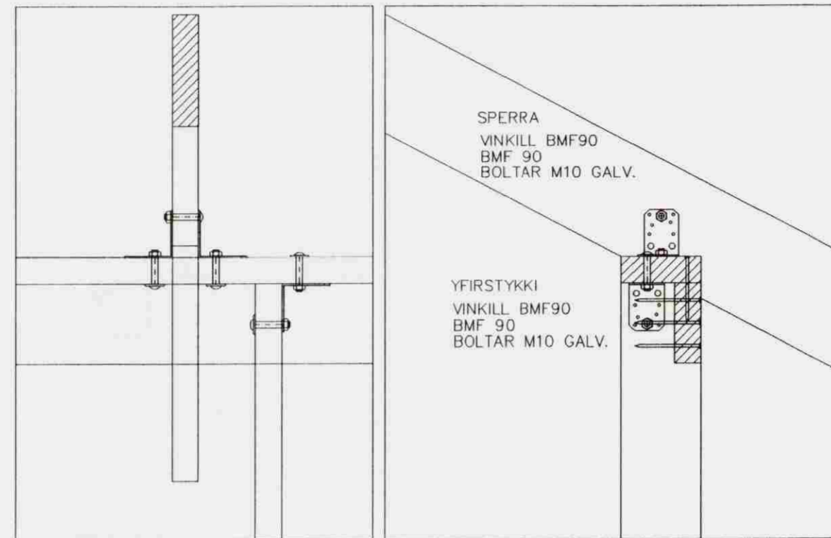
SÉRMYND FESTING SPERRA VIÐ SILLU
