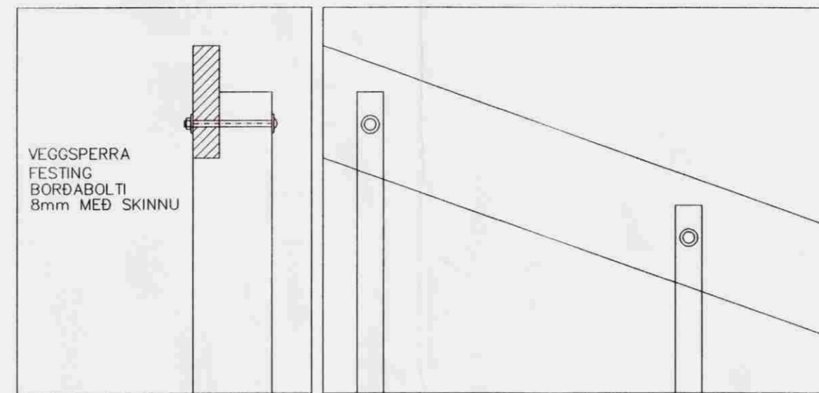
SÉRMYND SPERRA VIÐ ÚTVEGG (GAFL)
