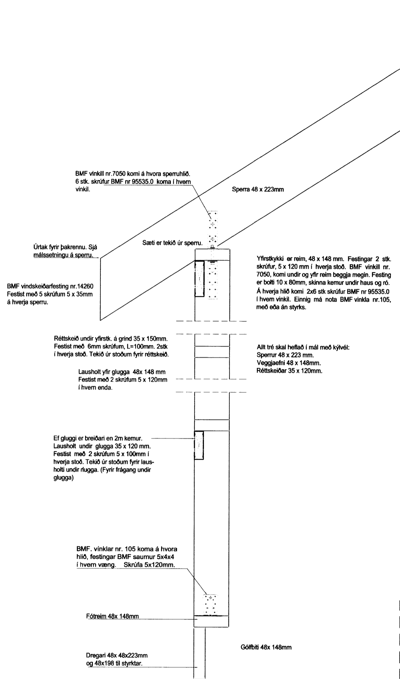
A SNIÐ - Almennt snið í útvegg. Mkv. 1:10
