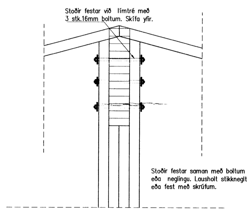
LÍMTRÉ MÖGULEG FESTING 1:10
