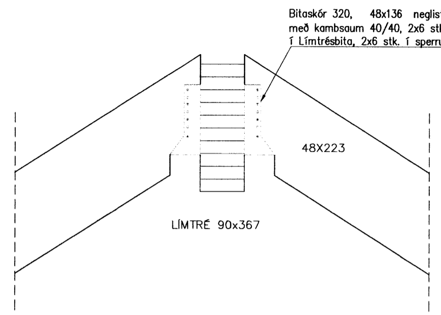
B Festing á sperrum í límtré. Mkv. 1:10
