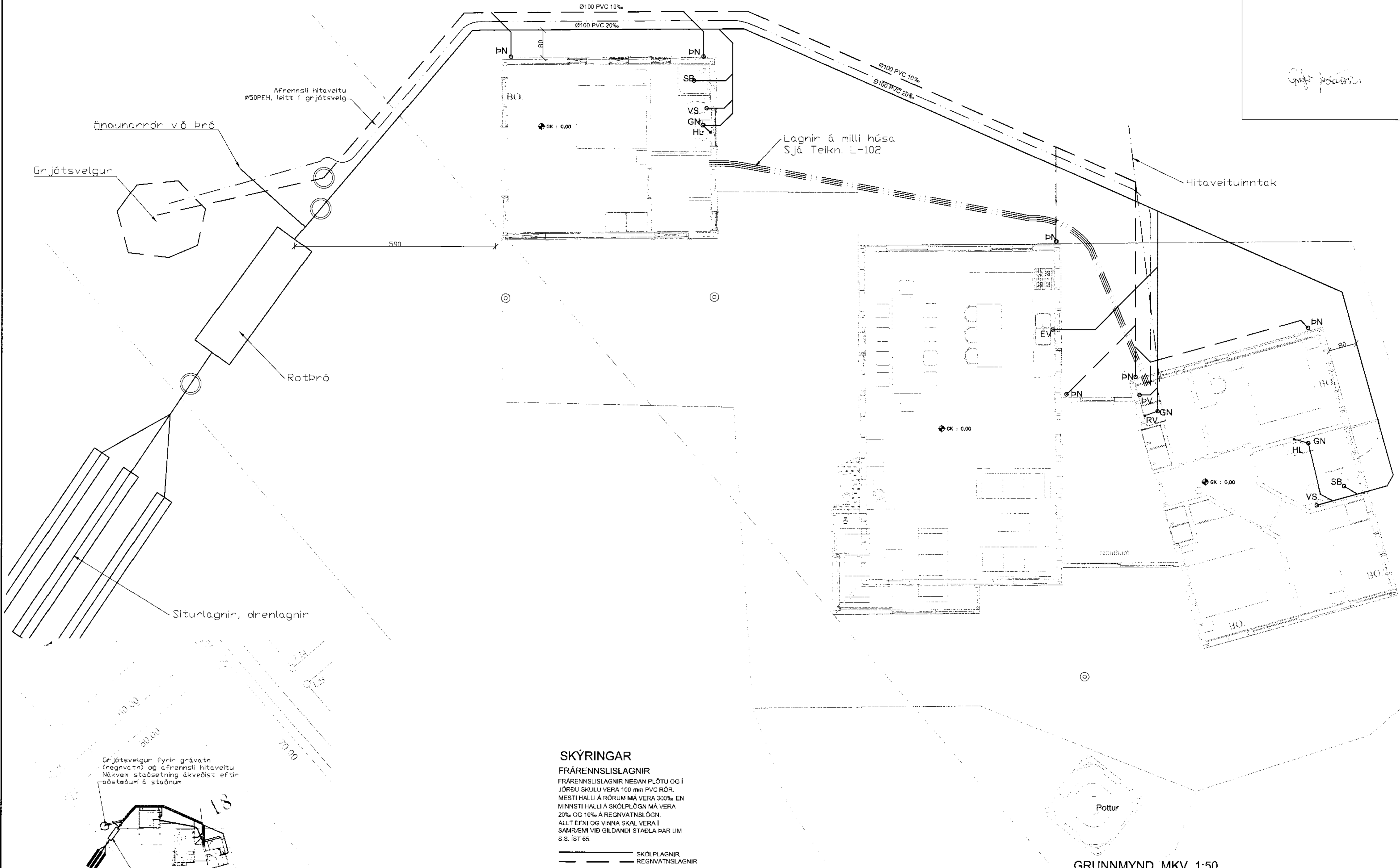
GRUNNMYND MKV. 1:50
