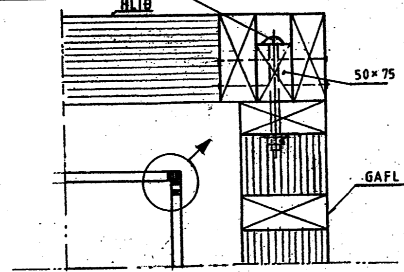
SAMSETNING Á HORNUM SÉÐ OFANFRÁ
