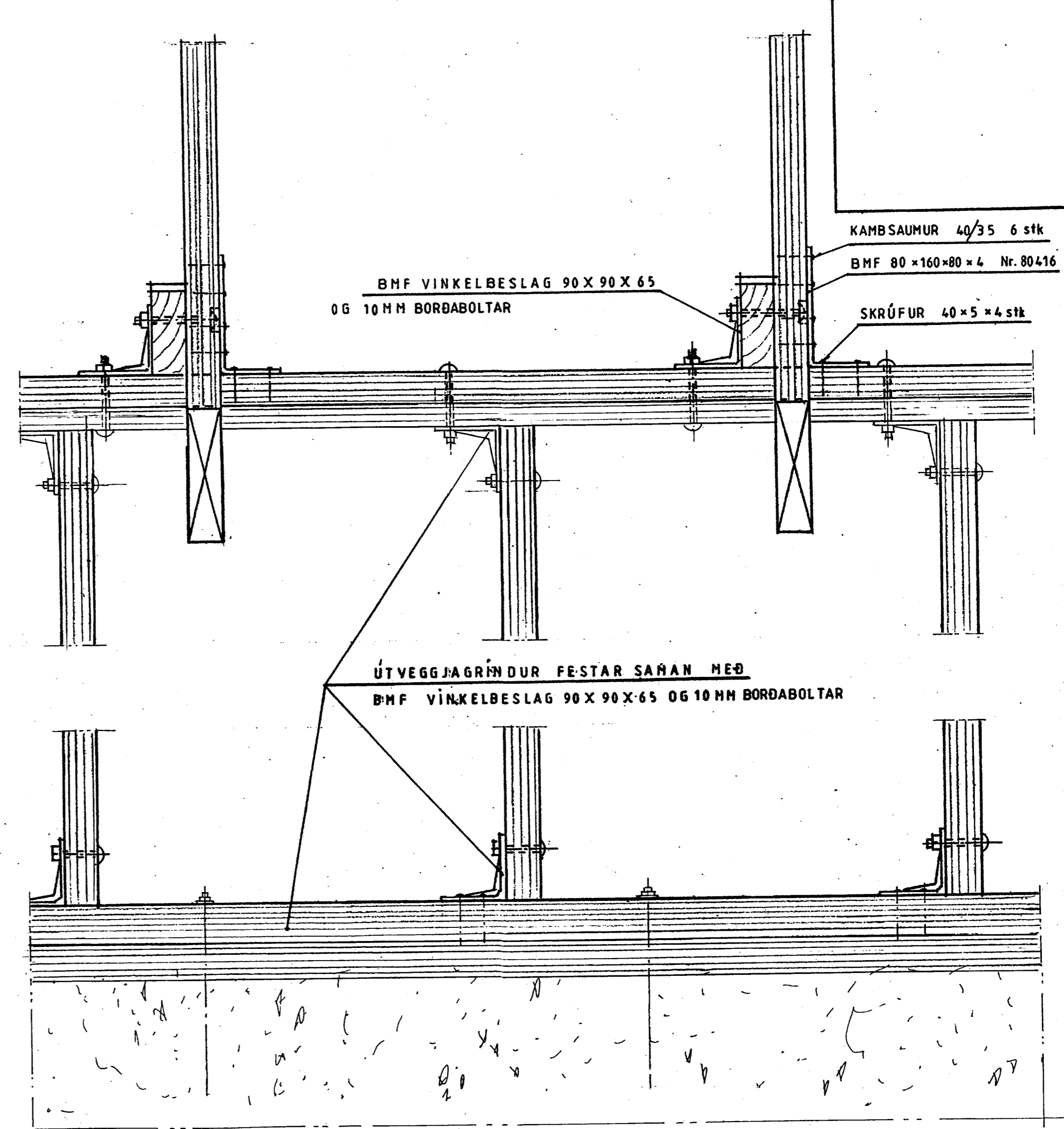
SÉÐ FRAMAN Á GRIND
