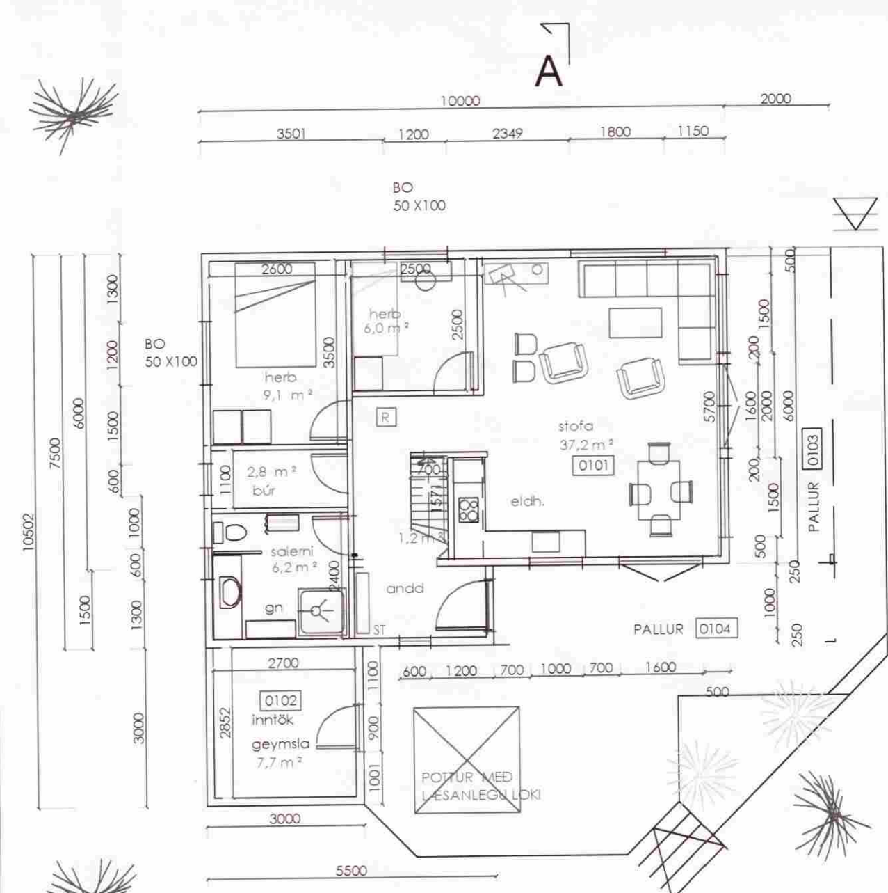
GRUNNMYND
