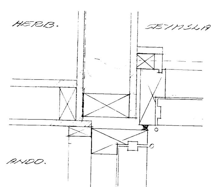
LÖBBÉTT SNIÐ VÍÐ INNGANG.
