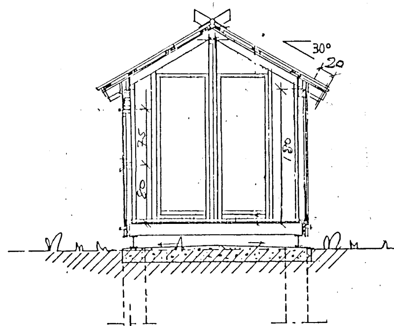
SNEIDMYND A-A.
