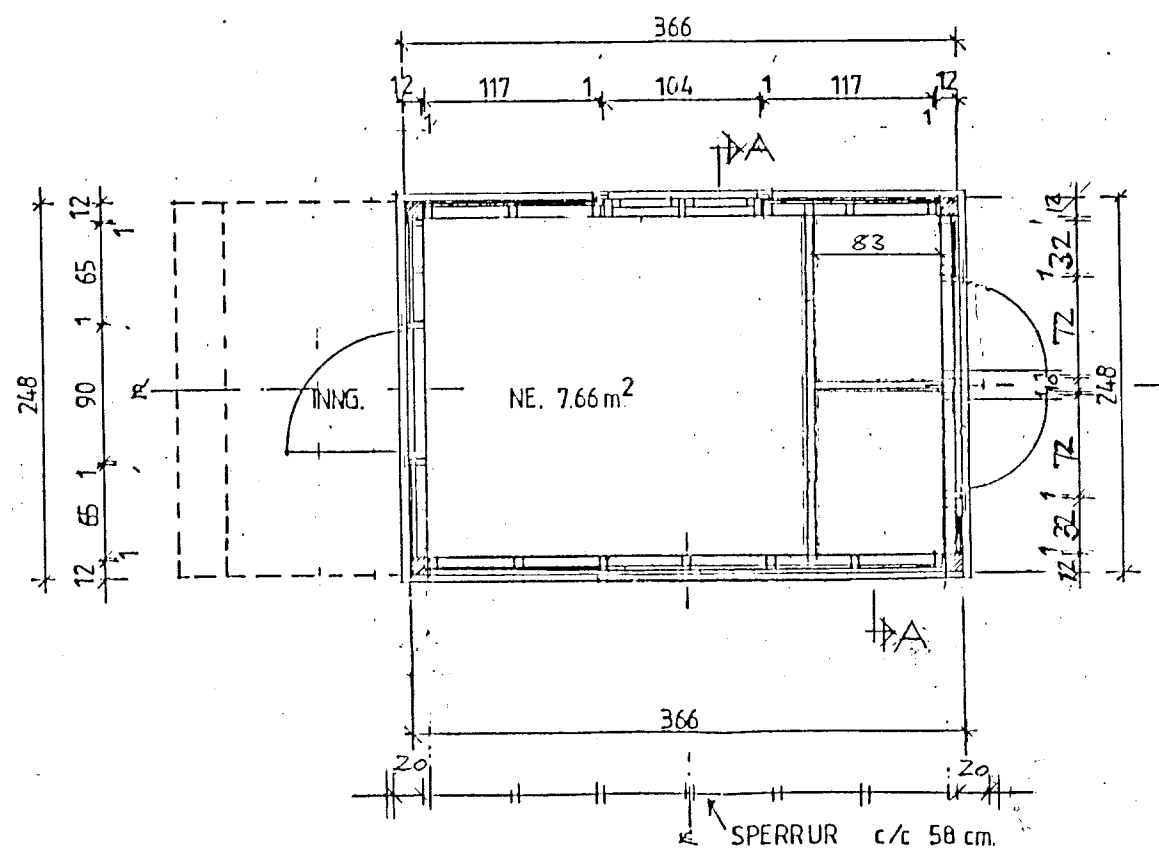
GRUNNMYND.
