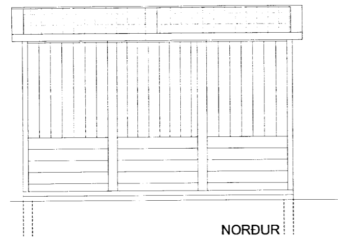
NORDUR M 1:50
