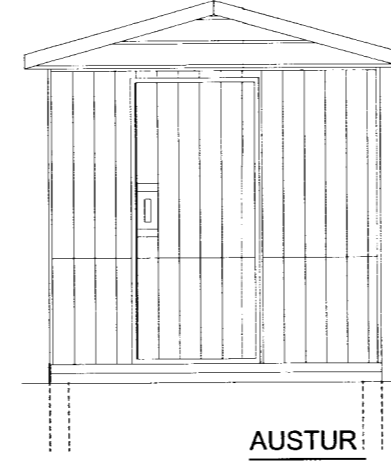
AUSTUR M 1:50
