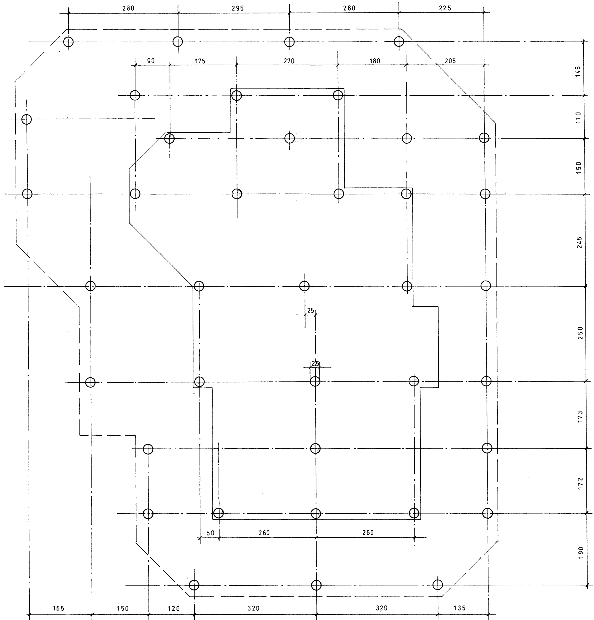
SÚLUUNDIRSÖÐUR, OFANVARP. Mkv.=1:50
