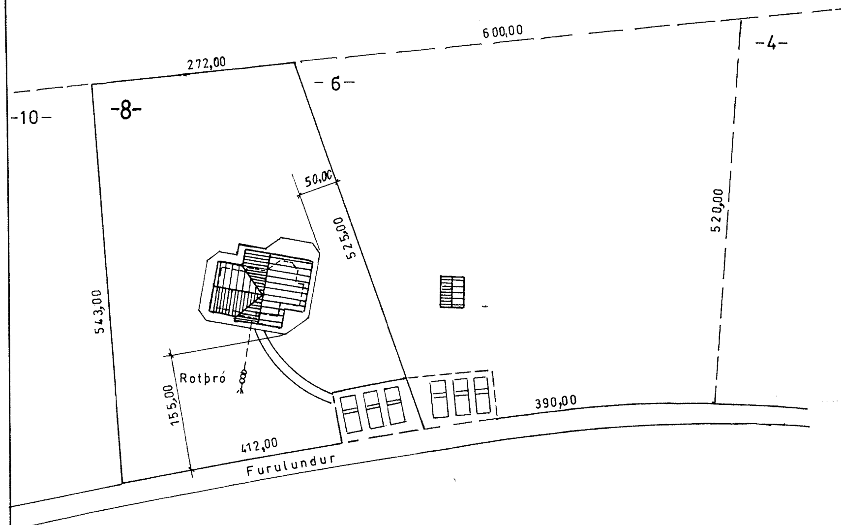
AFSTÖÐUMYND, Mkv.= 1:500
