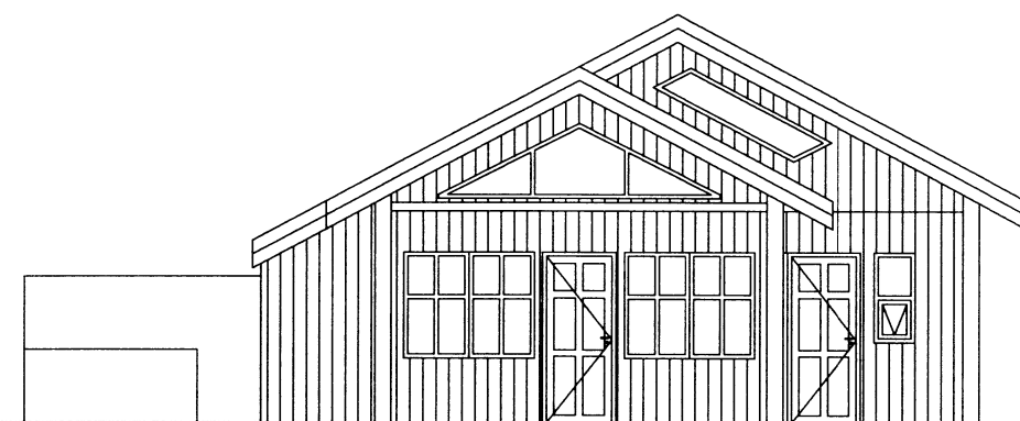
Útlit Mkv. 1:100
