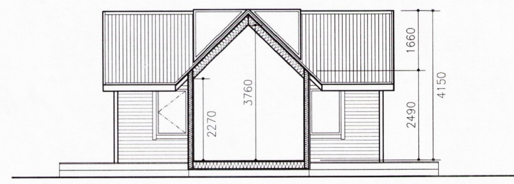
SNID A-A 1:100
