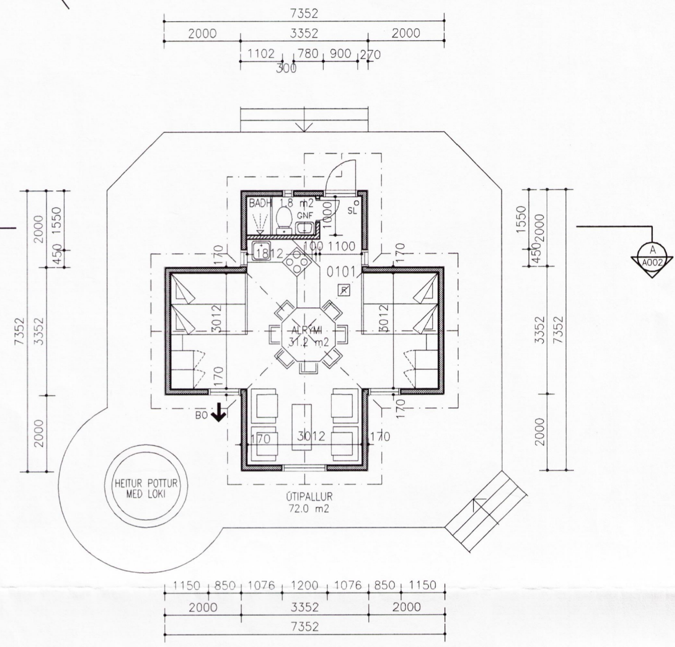
GRUNNMYND 1:100
