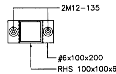
Sérmynd 1:3 1:10
