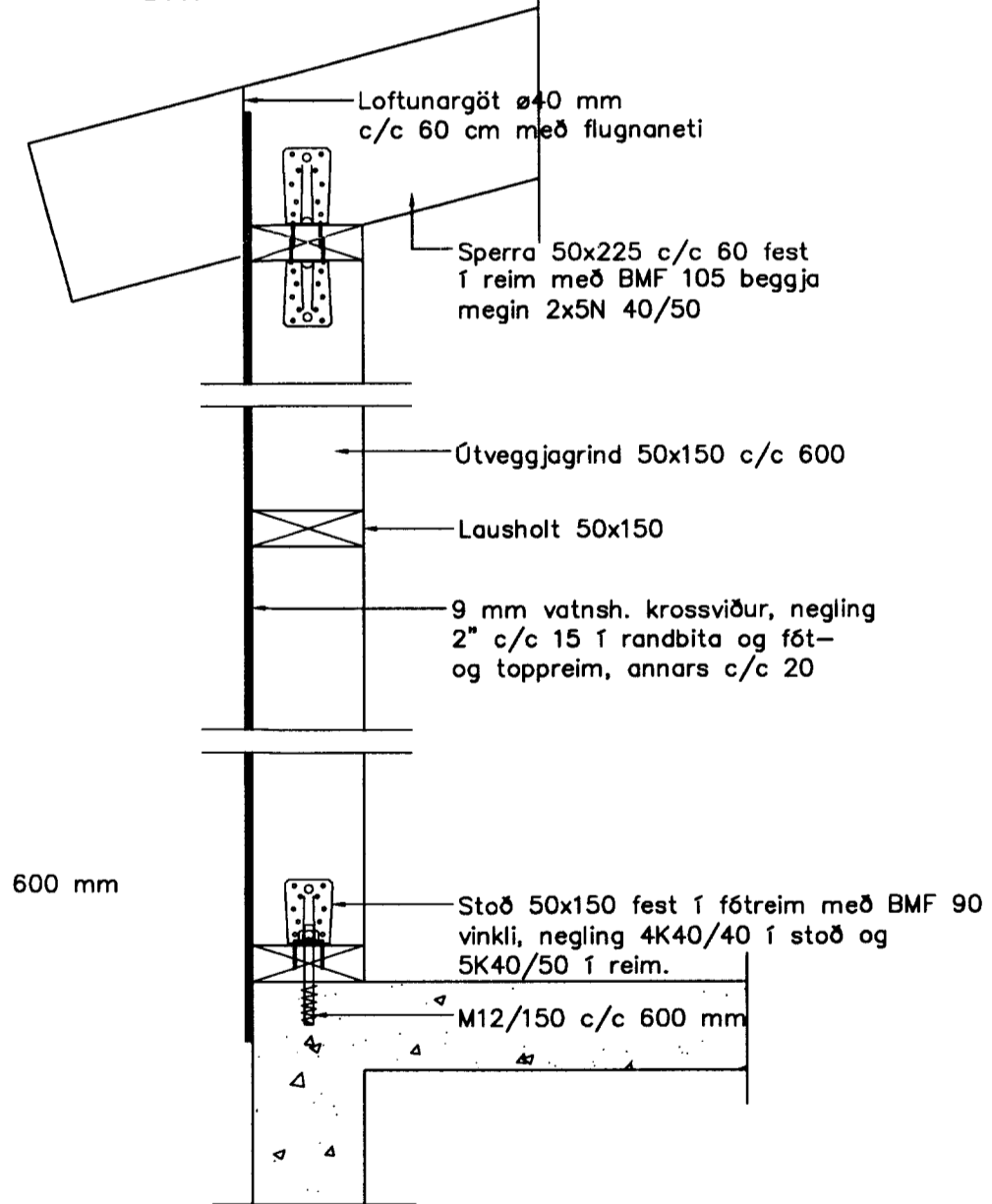
Snið I:I 1:10
