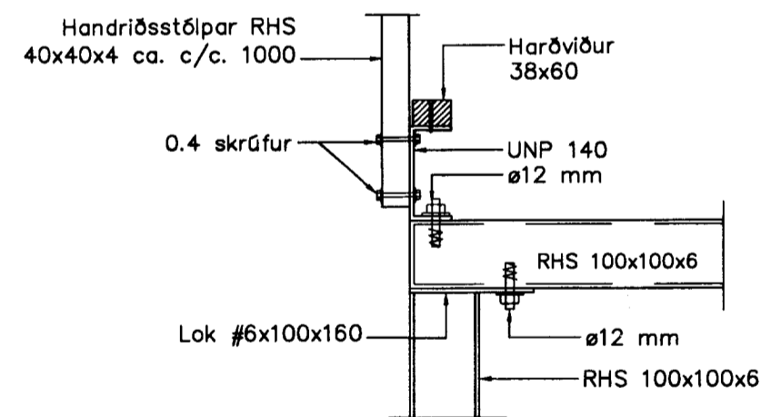
Sérmynd 1:4 1:10
