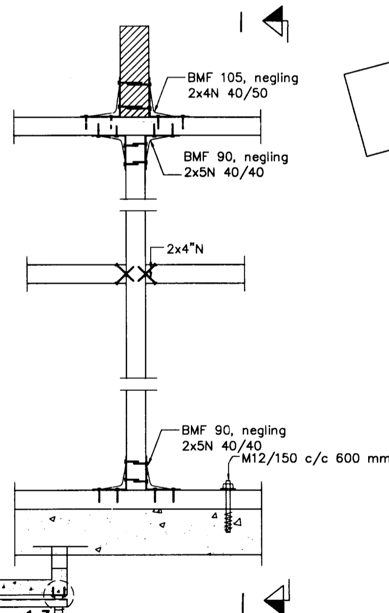
Sérmynd 1:1 1:10
