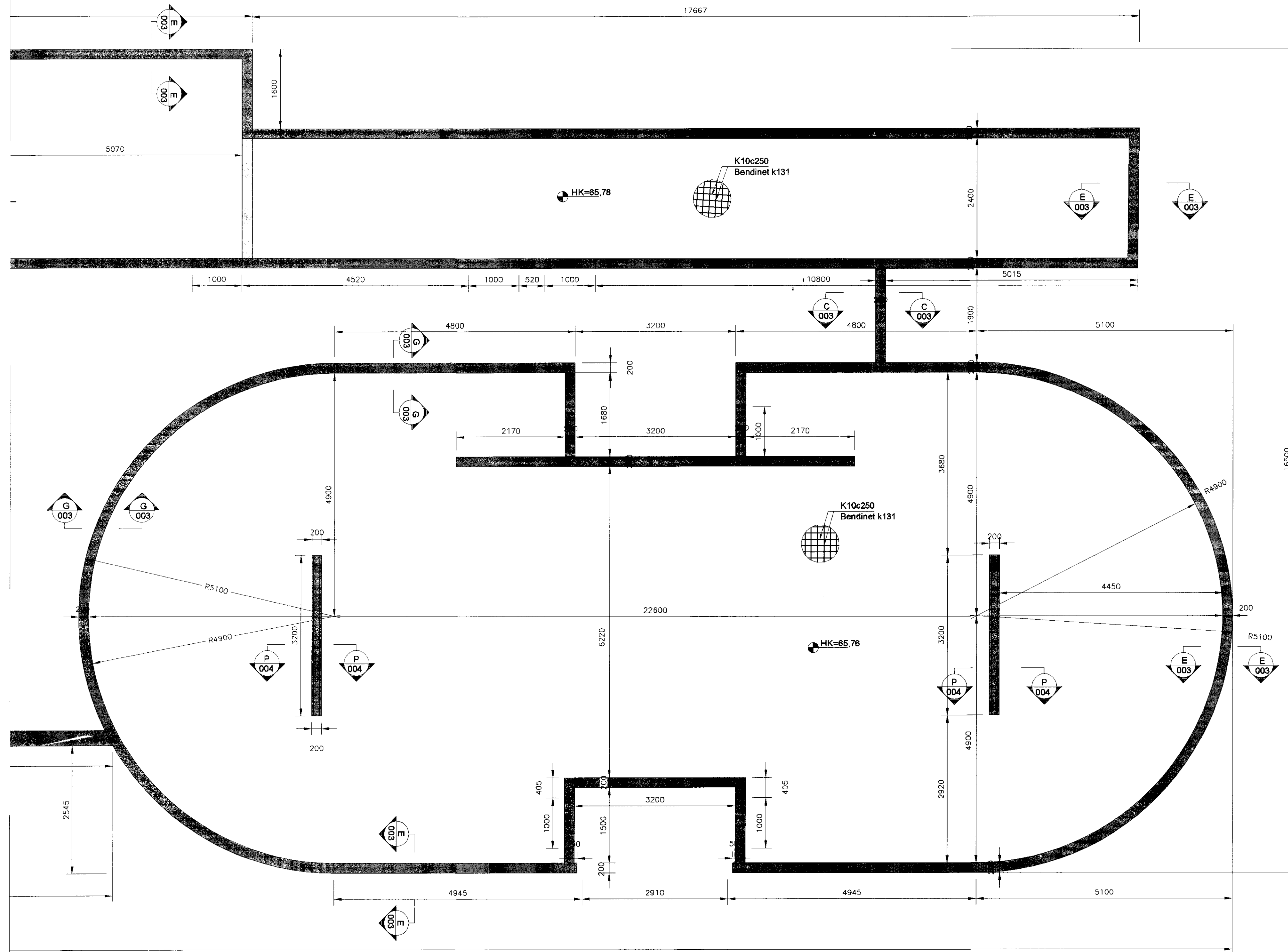
A SNID 002 1:20
