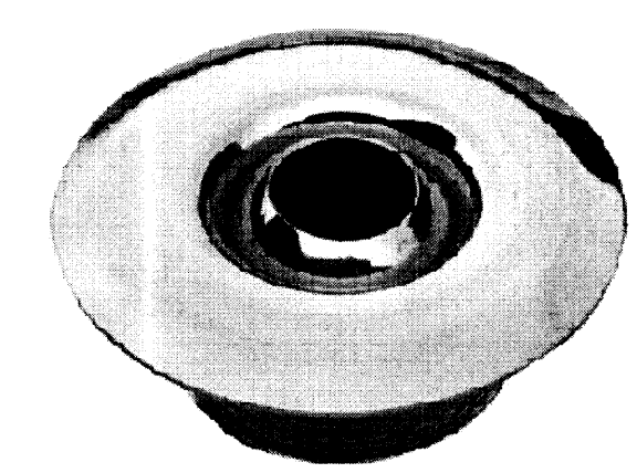
DÆMIGERÐUR INNRENNSLISSTÚTUR TENGING DN50, AFKÖST 2,25 l/s
