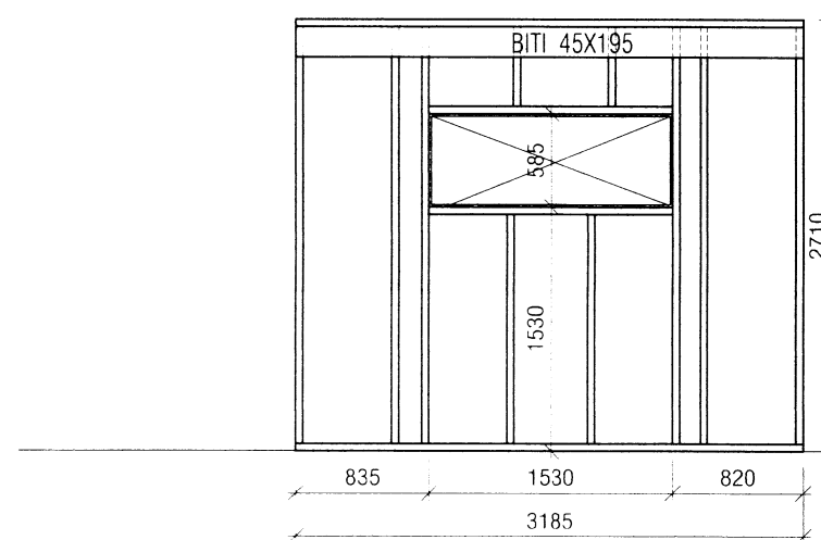
VEGGJA-GRIND, VESTUR
