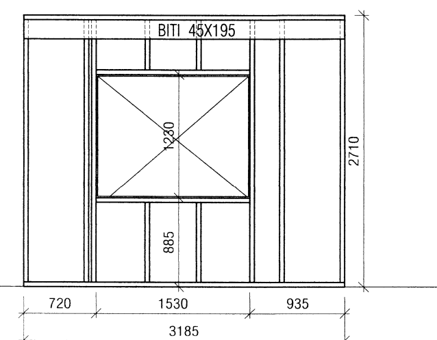
VEGGJA-GRIND, AUSTUR
