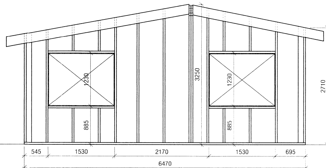
VEGGJA-GRIND, SUÐUR
