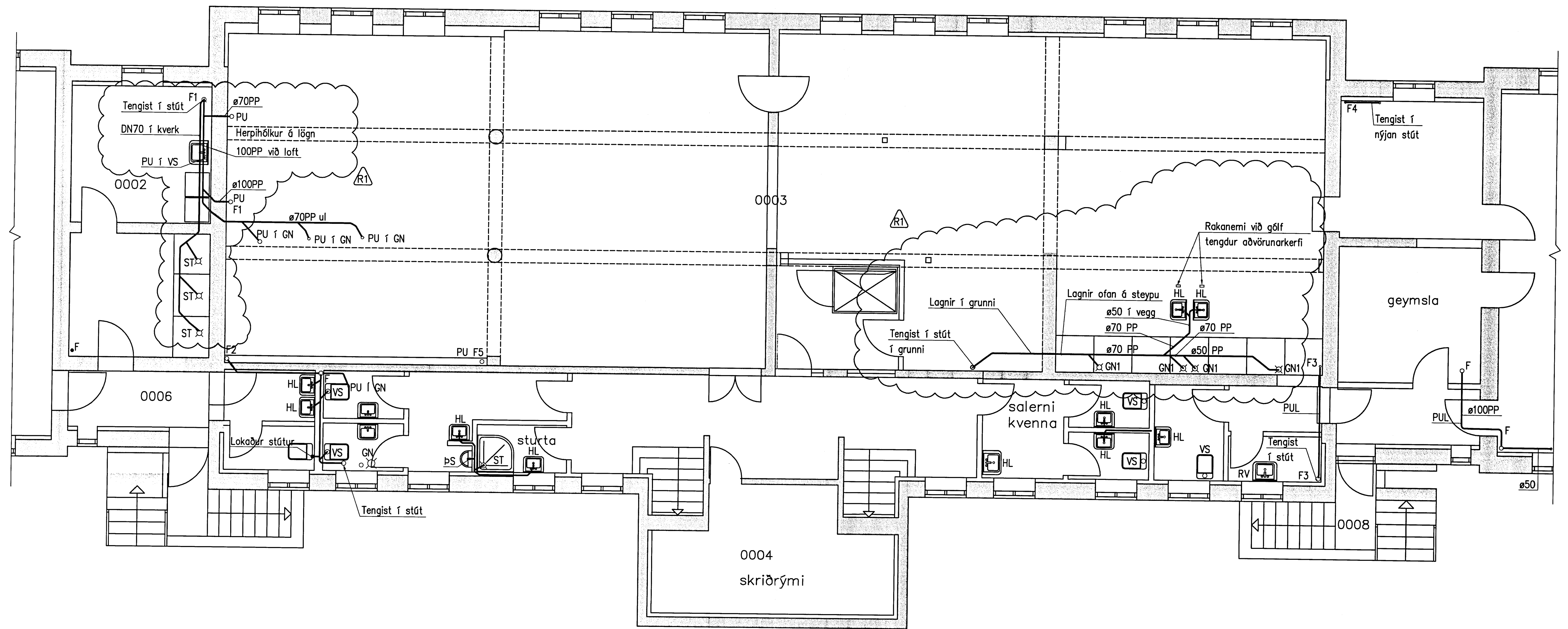
GRUNNMYND 1:50
