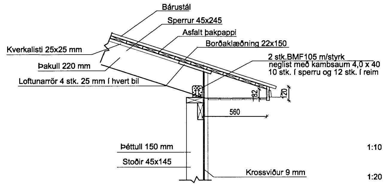
KENNISNIÐ 1:20
