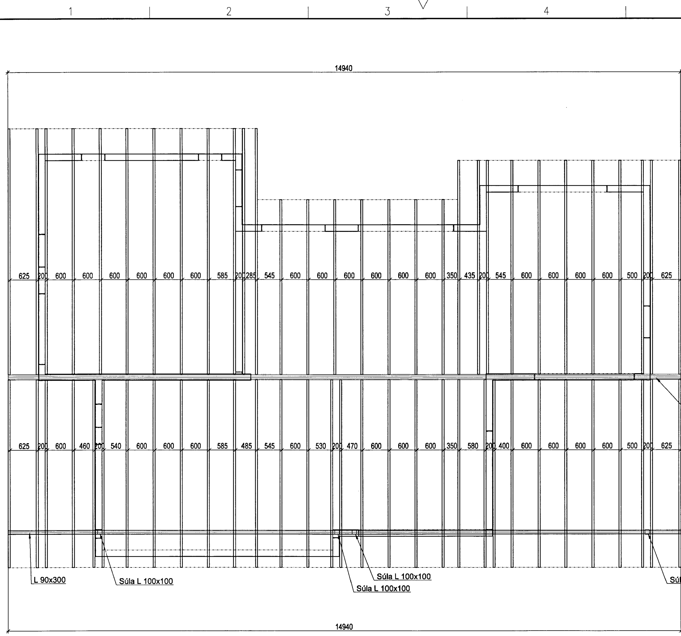
GRUNNMYND 1:50
