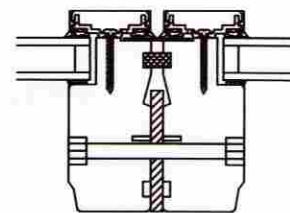
Lárétt deili Ísteypt stálfesting og samsetning glugga. Gluggaþingir boltaðar saman með 10 mm borðaboltum, þétt með ull, límdri tré- fjóður og álfasningu. Mkv. 1:5
