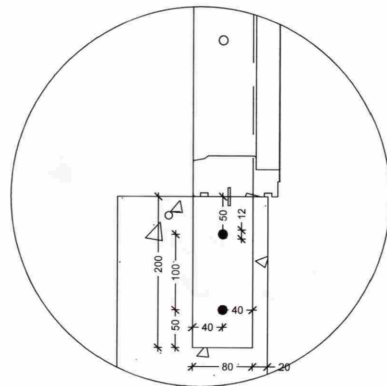
Lóðrétt deili Ísteypt stálfesting járnþent með K10 í sökkli og boltað við glugga með borðaboltum Mkv. 1:5
