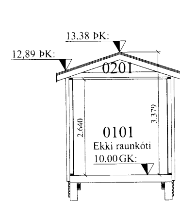
SNÍÐ B-B
