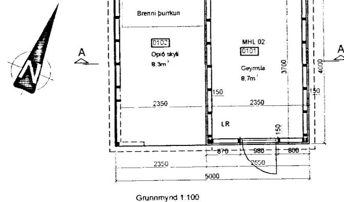
Grunnmynd 1:100
