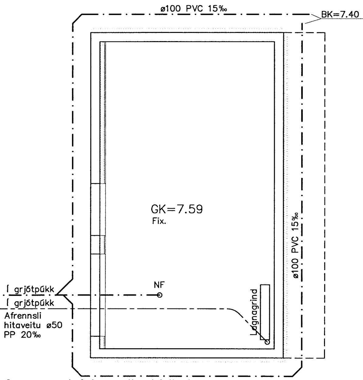
Grunnmynd frárennsli -kjallari Mkv. 1:50
