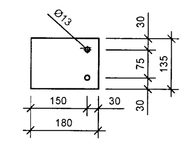
STÁLPLATA S1 t=10mm
