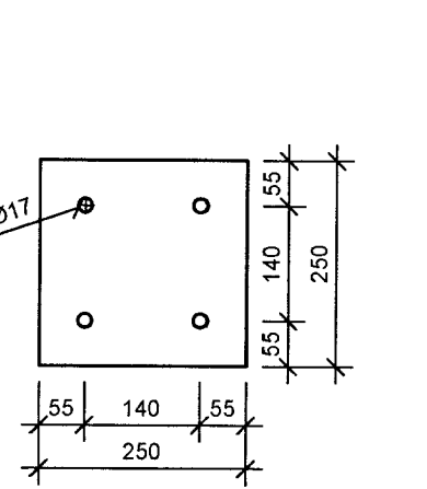
STÁLPLATA S6 t=15mm
