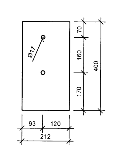
STÁLPLATA S4 t=10mm
