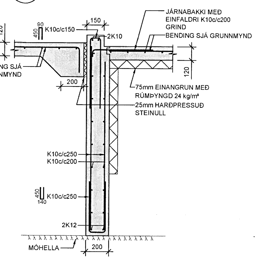
20 SNID 1:20 B-101
