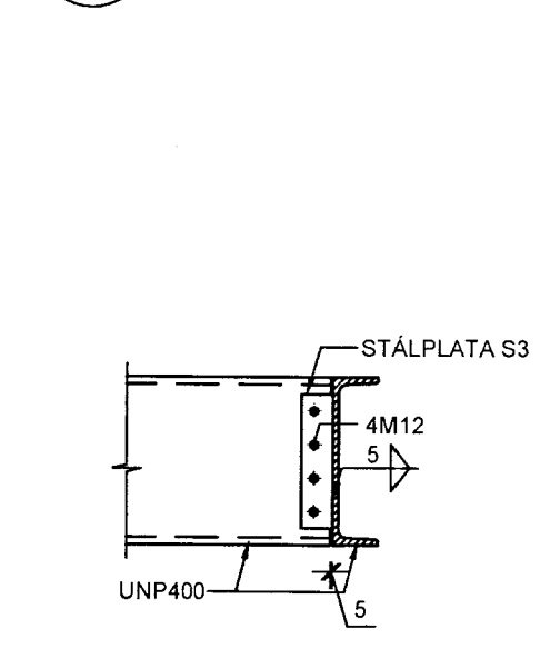
15 SNID 1:20 B-101
