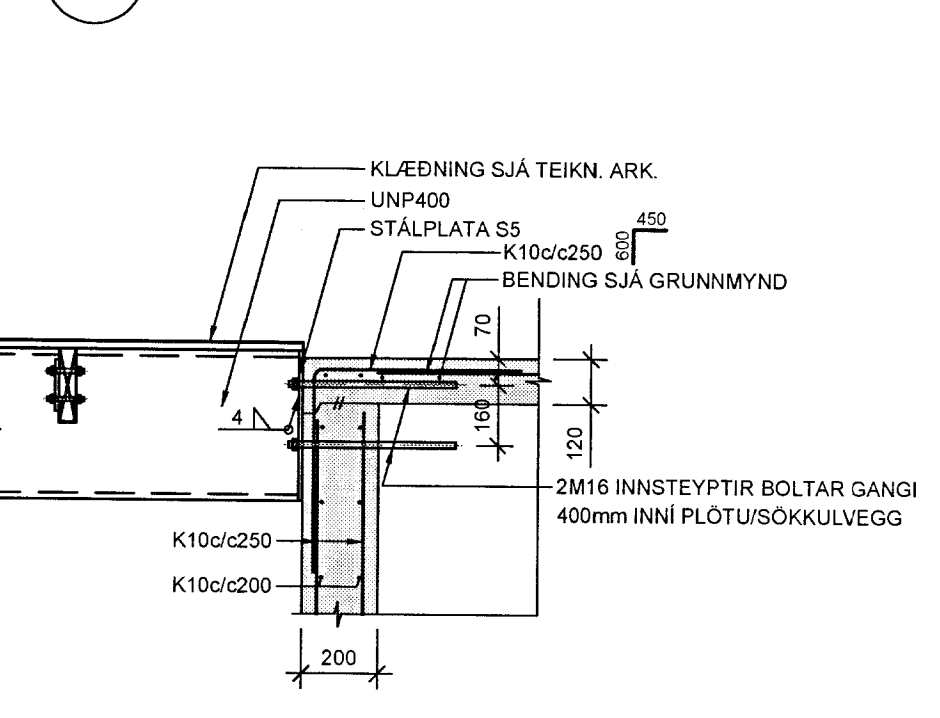
18 SNID 1:20 B-101
