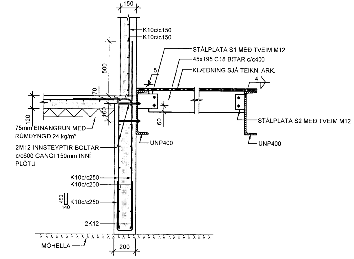
14 SNID 1:20 B-101
