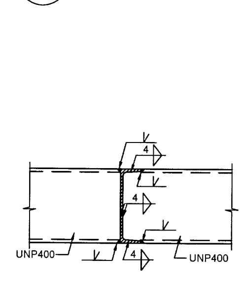
16 SNID 1:20 B-101
