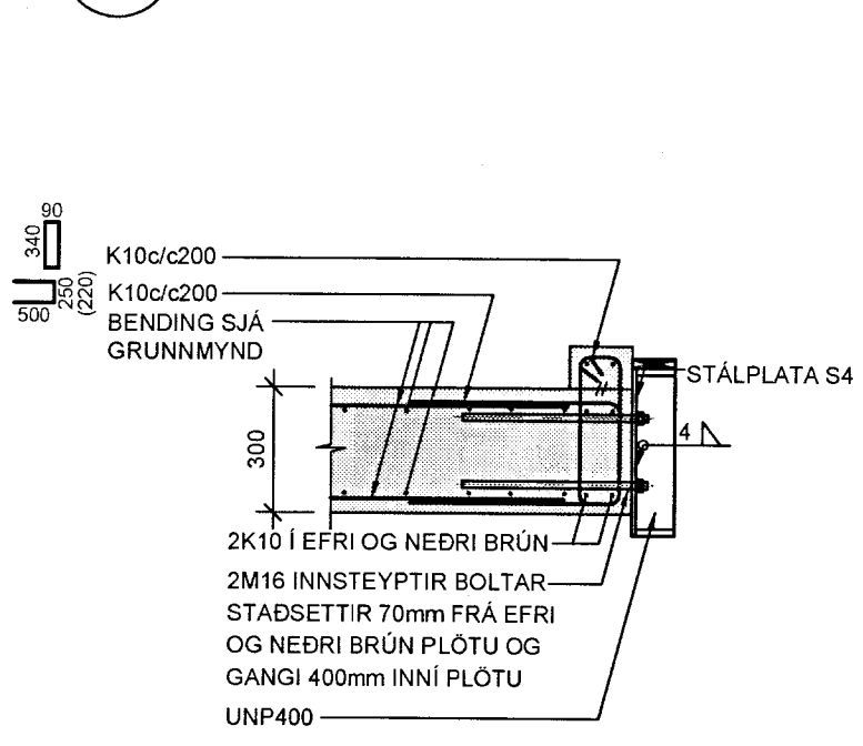
17 SNID 1:20 B-101
