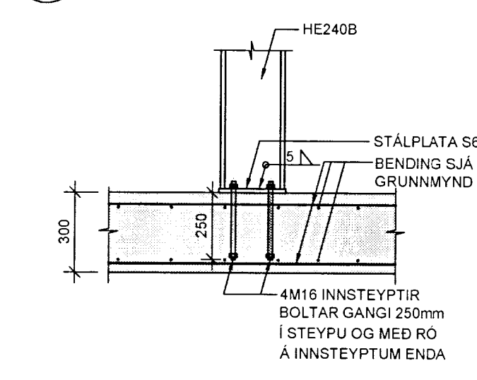
19 SNID 1:20 B-101
