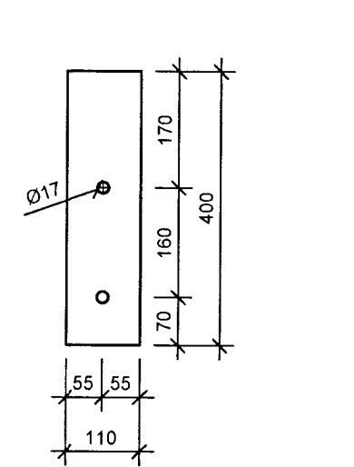
STÁLPLATA S5 t=10mm
