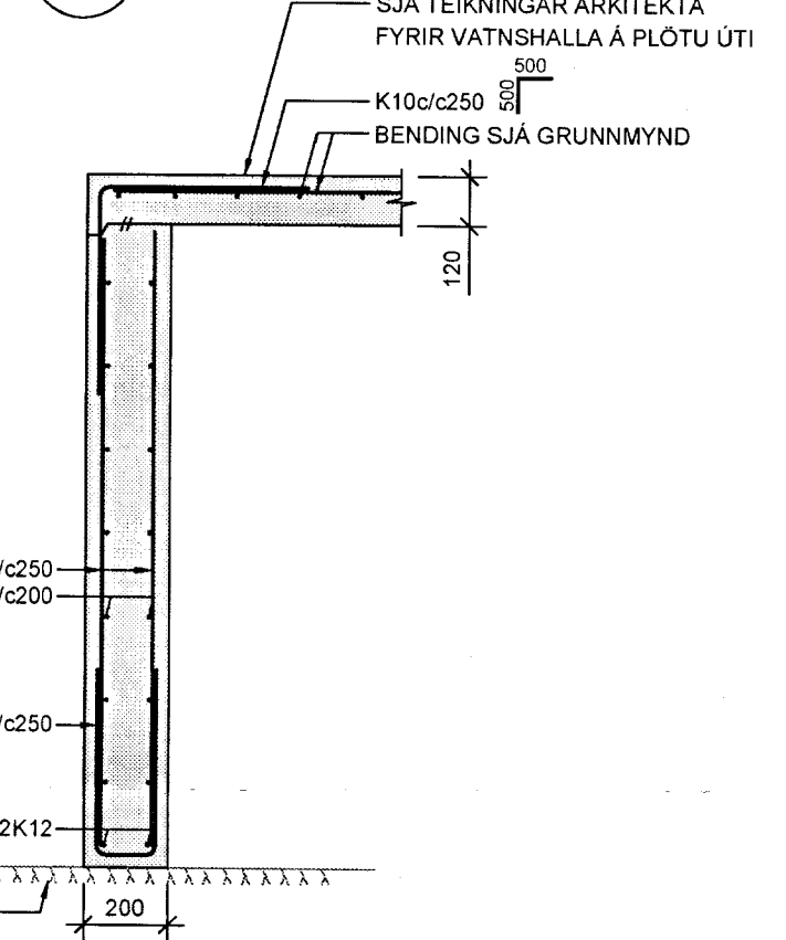
21 SNID 1:20 B-101
