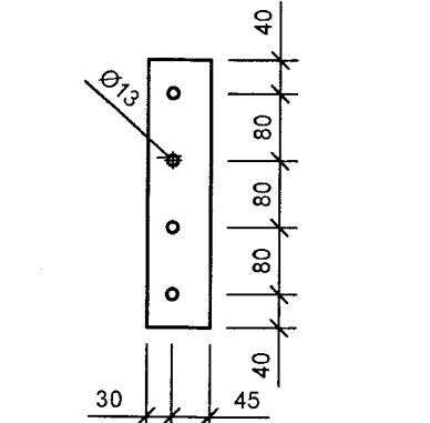
STÁLPLATA S3 t=10mm
