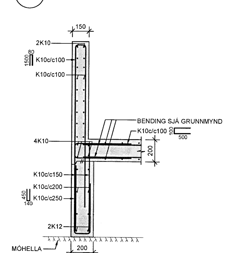
23 SNID 1:20 B-101
