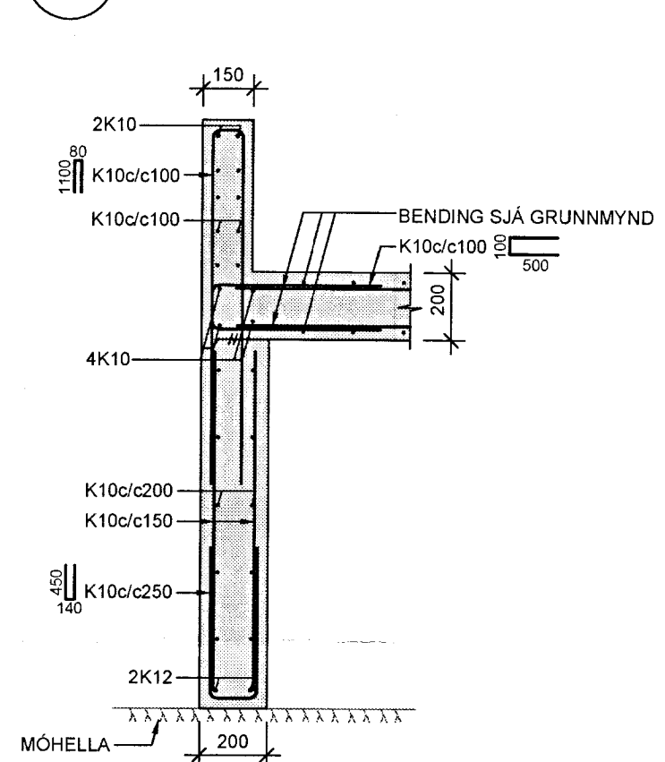
22 SNID 1:20 B-101
