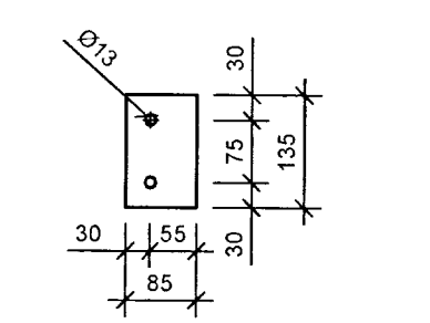
STÁLPLATA S2 t=10mm
