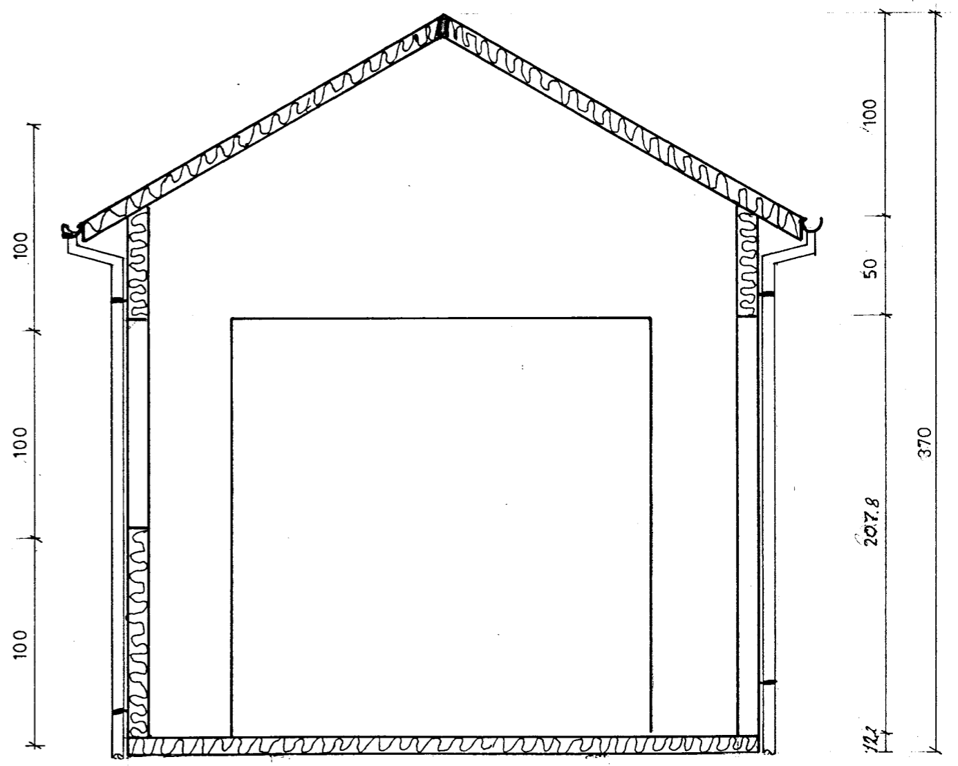
SNEÐ. AA
