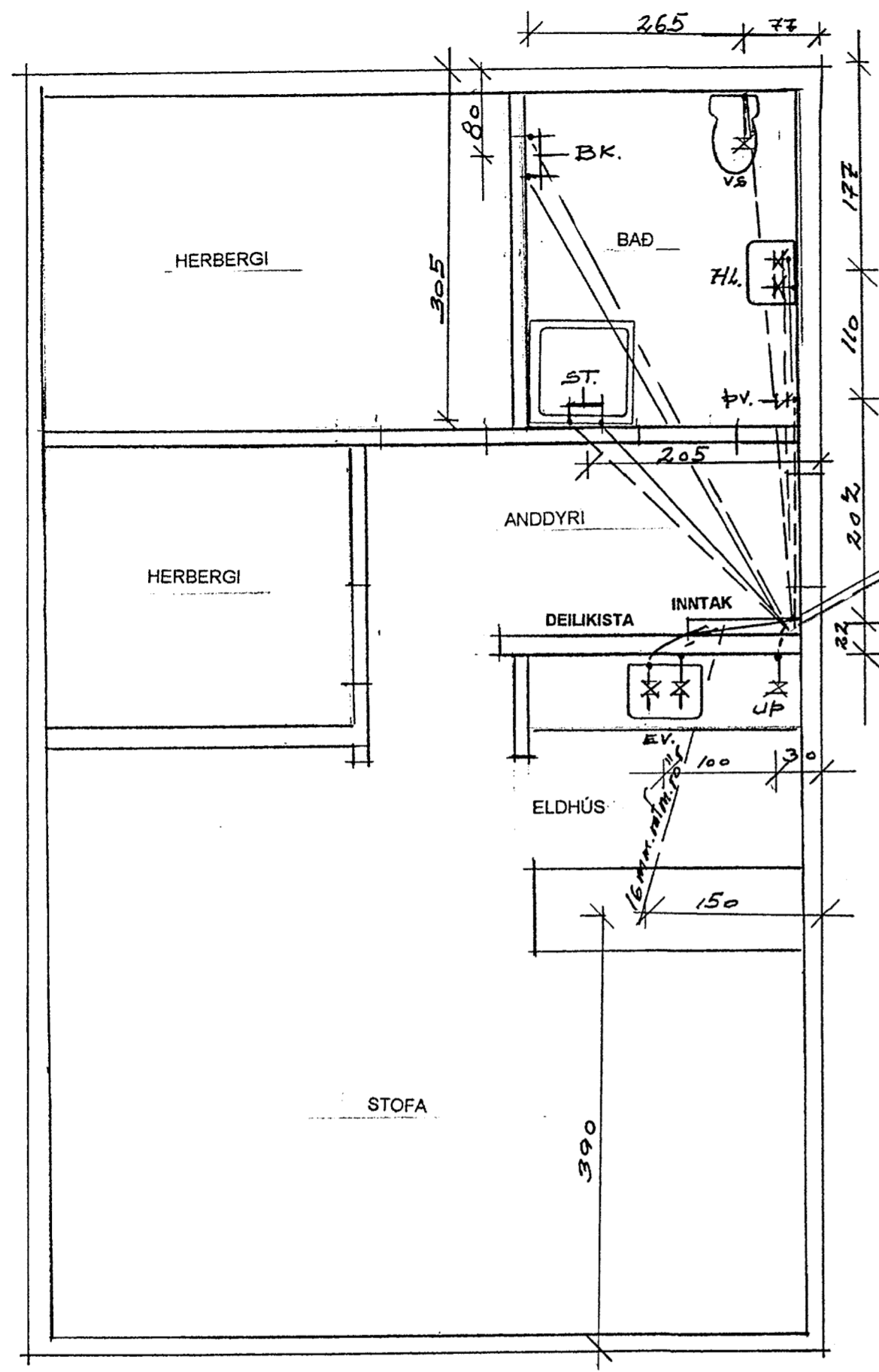
GRUNNMYND ÍBÚÐ 1:50
