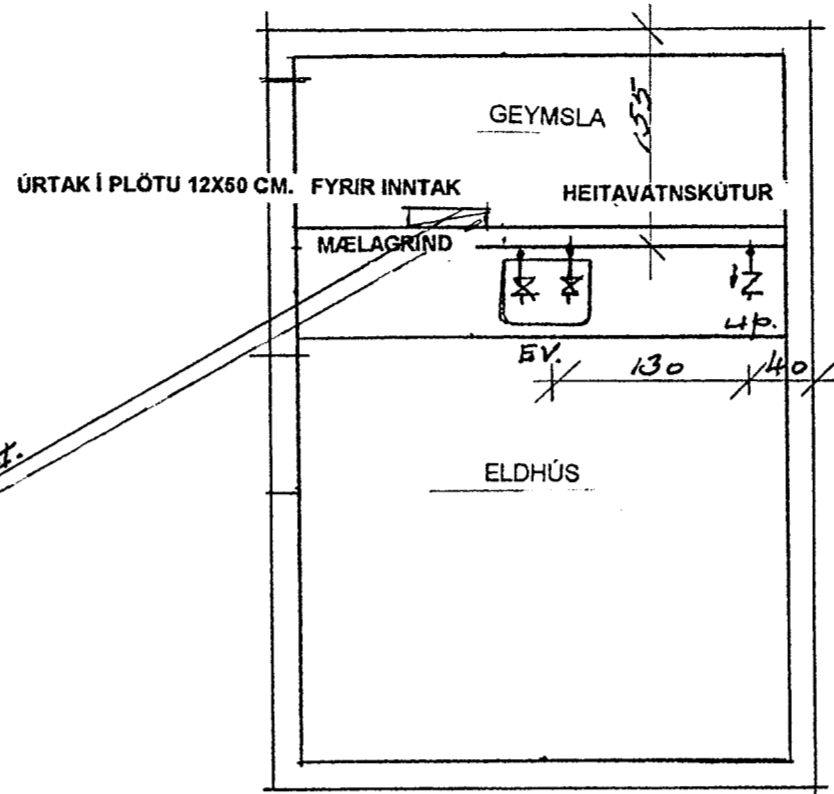
GRUNNMYND GESTAHÚS 1:50
