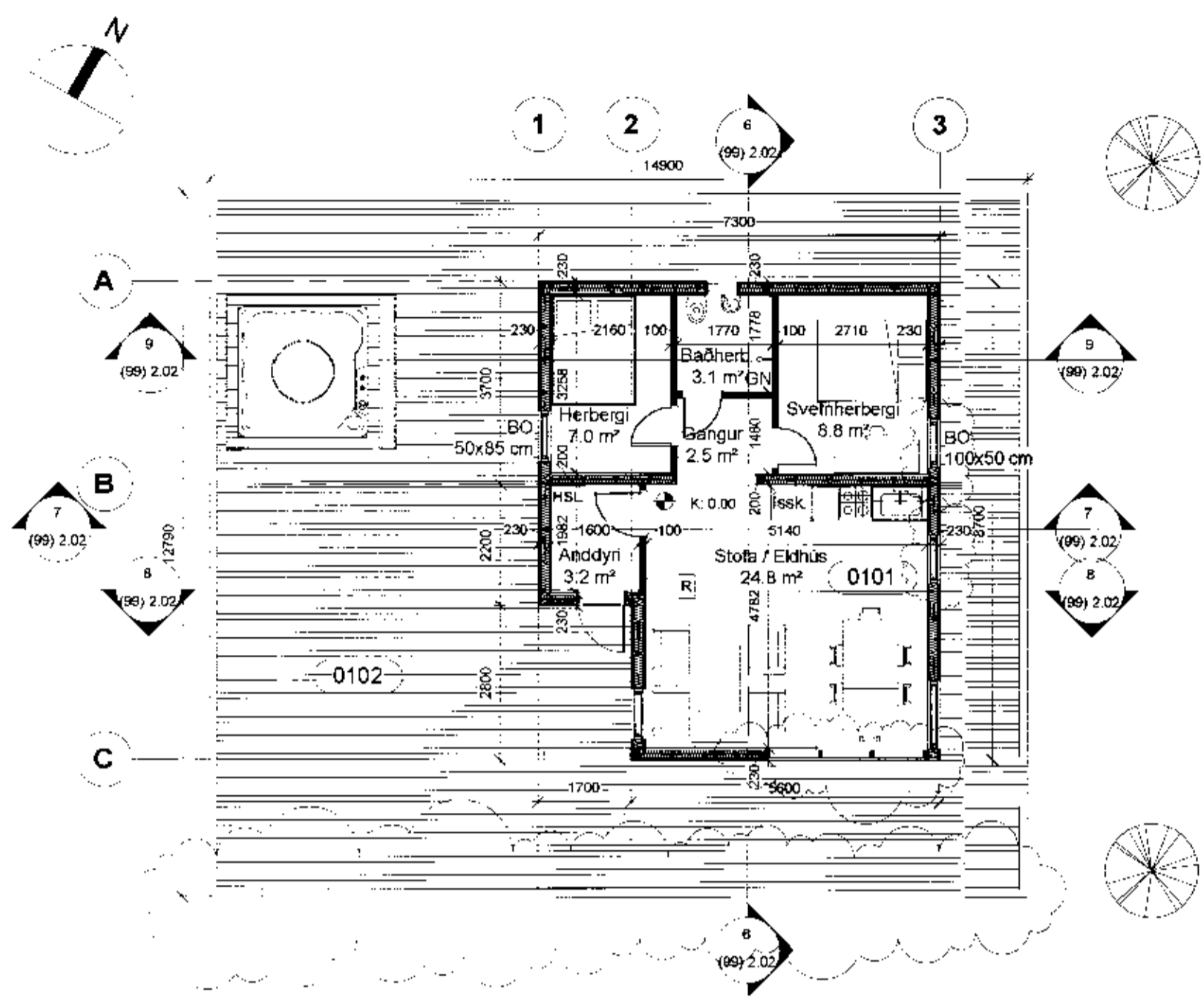
1 Grunnmynd 1. hæð 1 : 100
