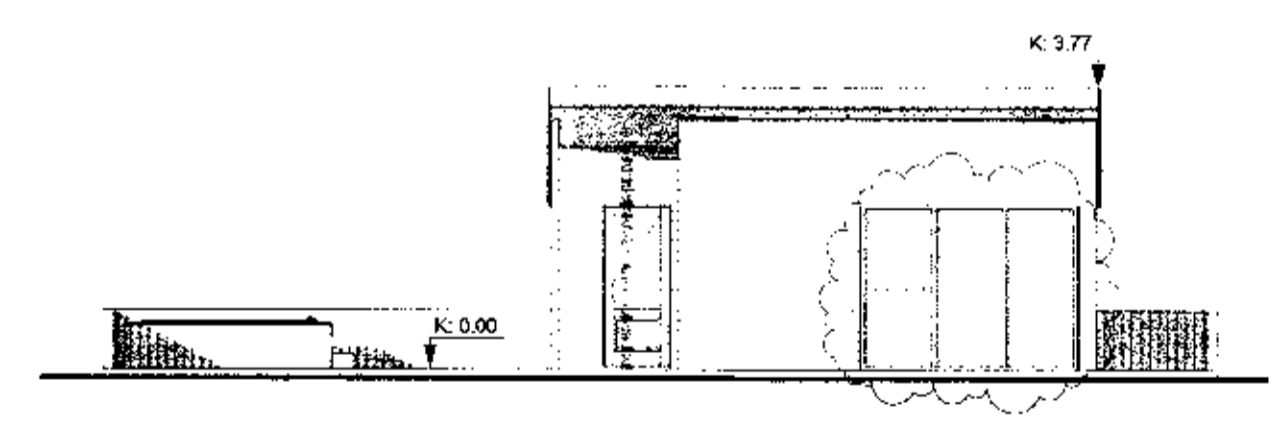
5 Ásýnd suður 1 : 100
