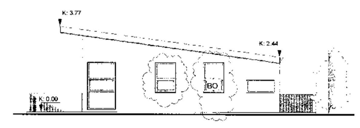
2 Ásýnd austur 1 : 100
