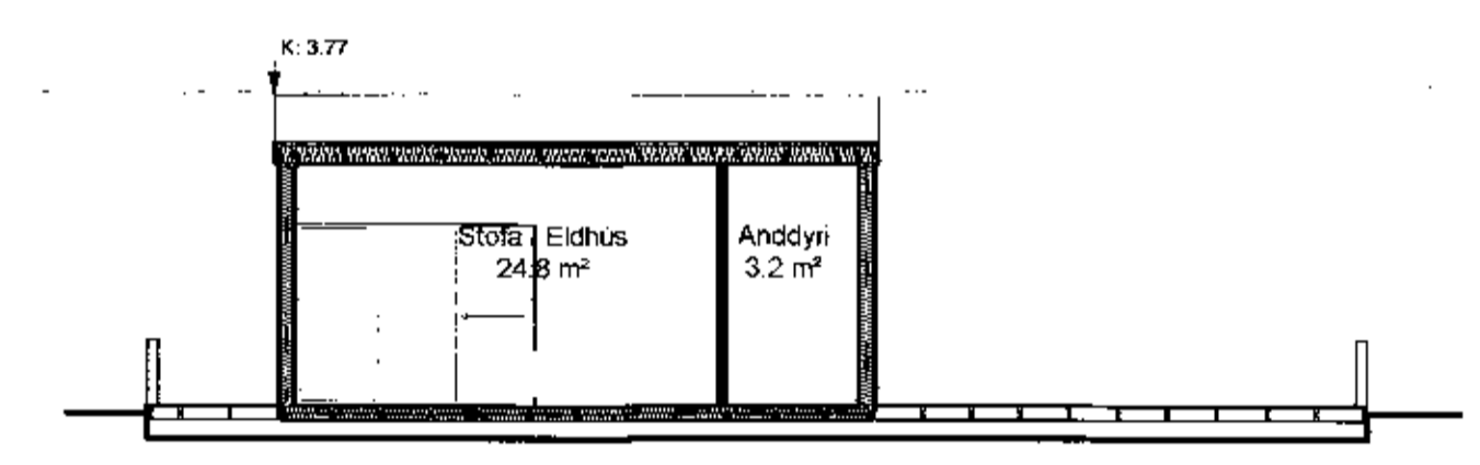
8 Sneiðing C-C 1 : 100
