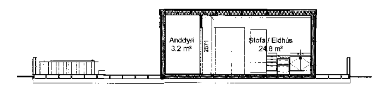
7 Sneiðing B-B 1 : 100
