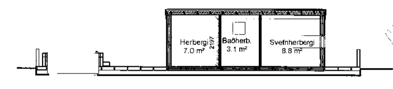
9 Sneiðing D-D 1 : 100
