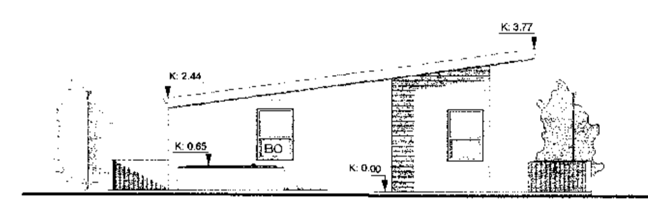
3 Ásýnd vestur 1 : 100
