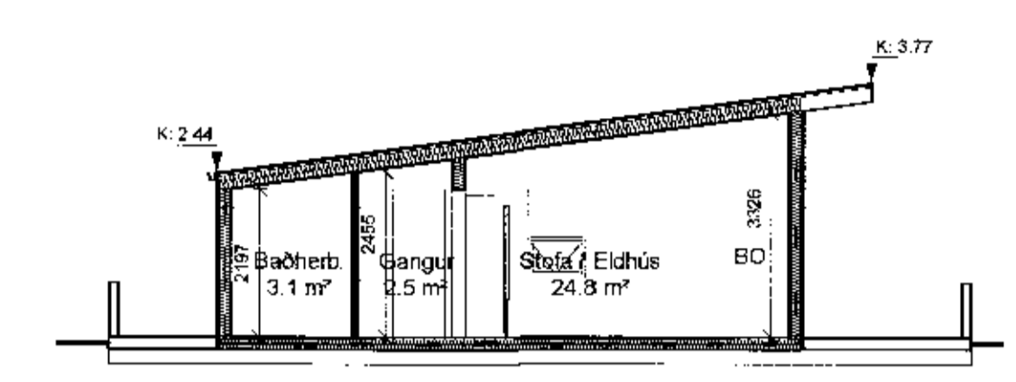
6 Sneiðing A-A 1 : 100
