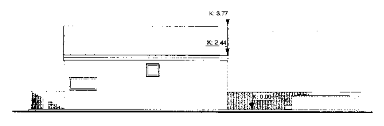
4 Ásýnd norður 1 : 100
